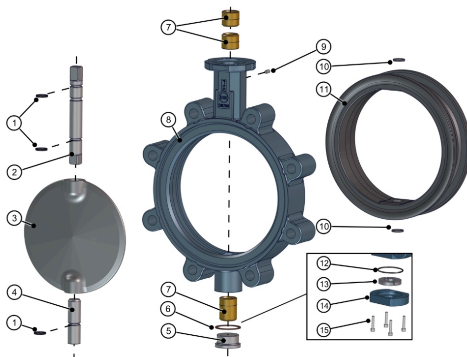
Fig. 15: Listă de componente Z014-A
