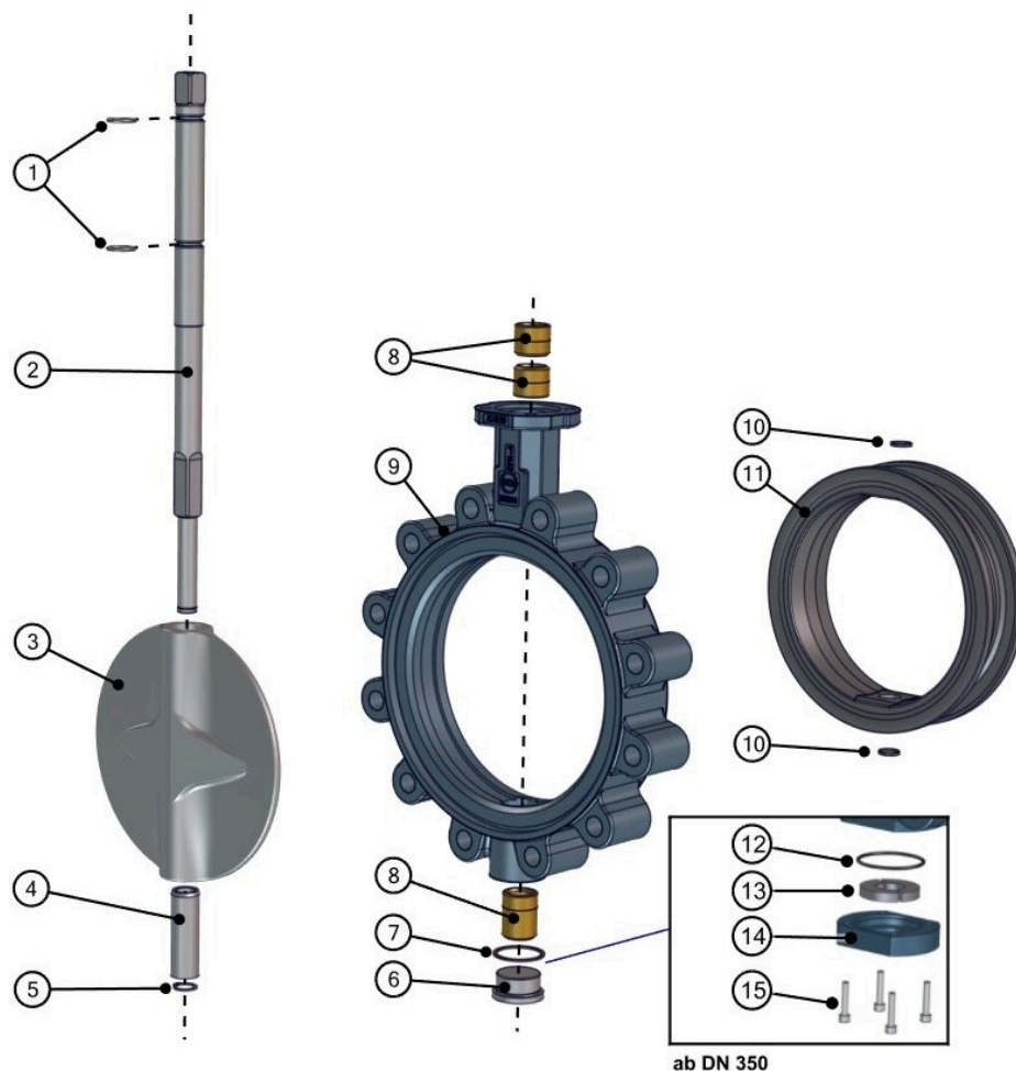
Fig. 16: Listă de componente Z014-A arbore TS
