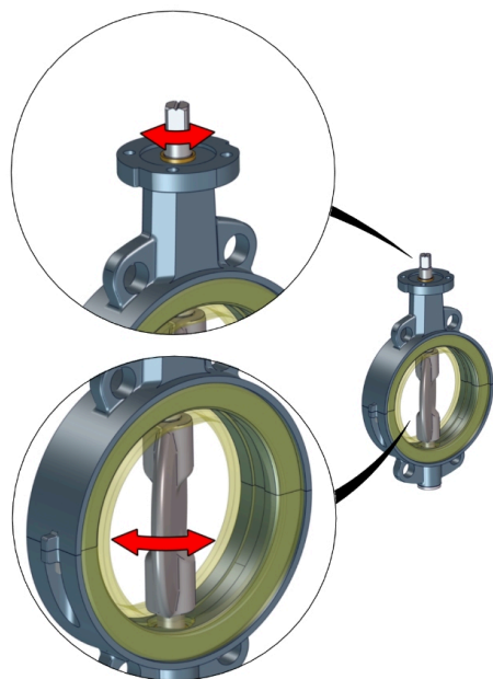
Fig. 4: Piese mobile
