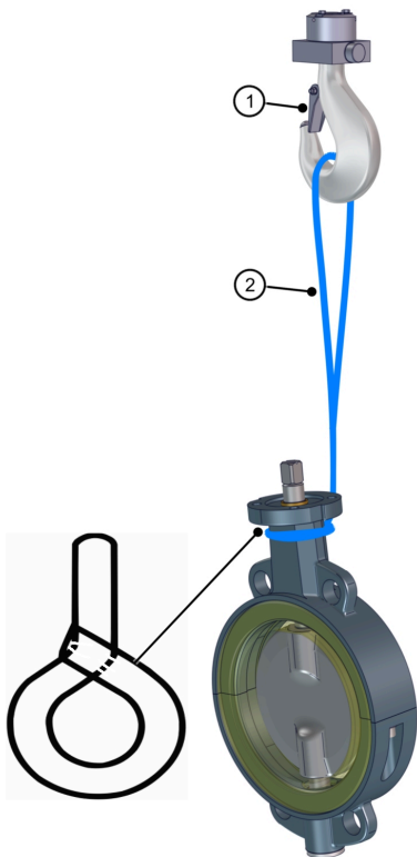
Fig. 6: Ridicarea clapetei interpusă între flanșe cu macaraua
