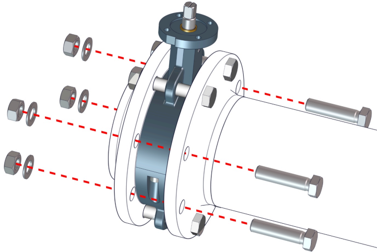
Fig. 9: Înșurubați clapeta interpusă între flanșe
