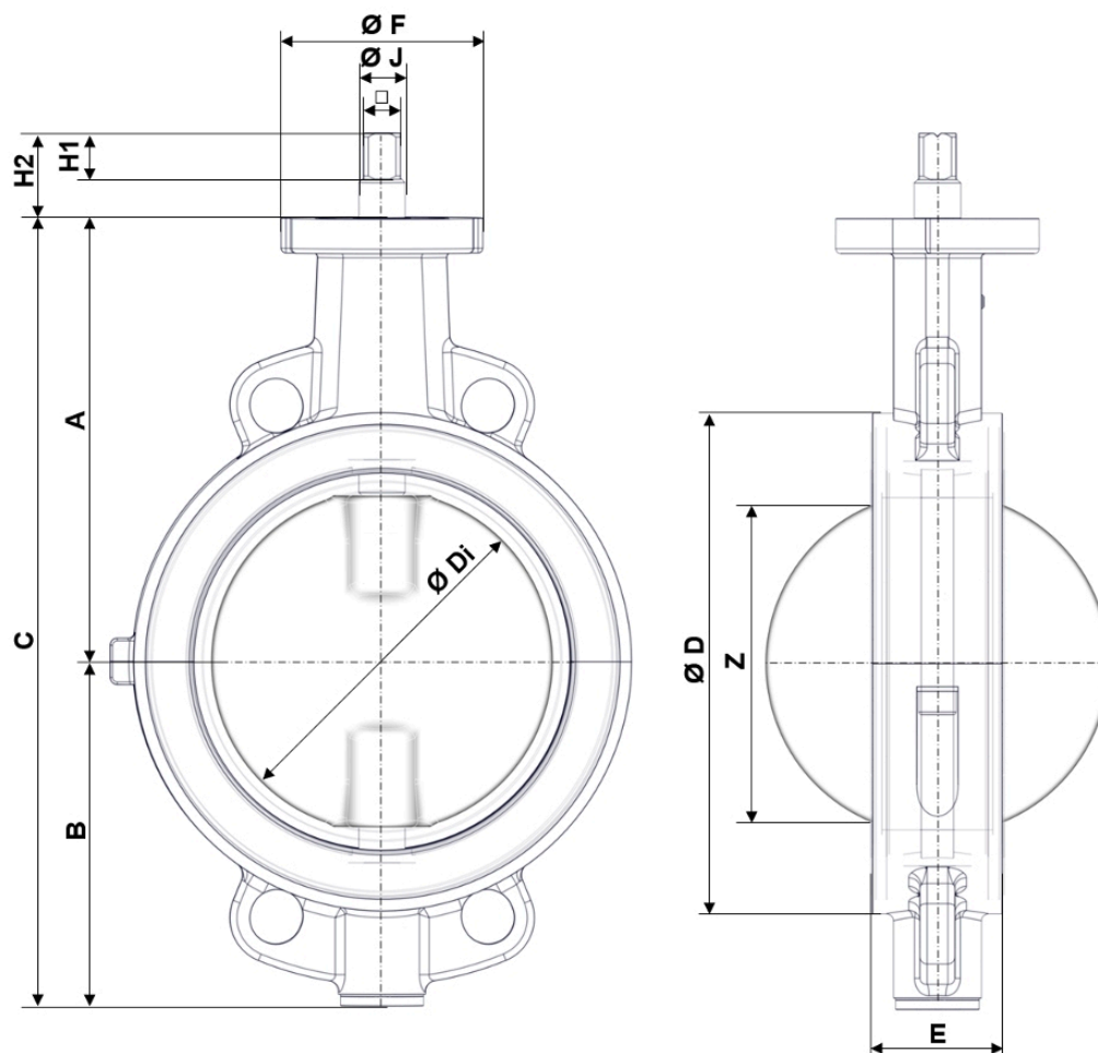
Fig. 3: Dimensiuni principale Z011-GMX
