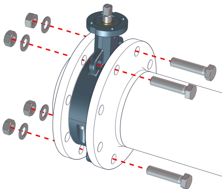
Fig. 8: Poziționați clapeta interpusă între flanșe
