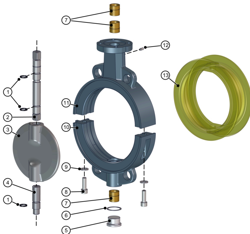
Fig. 15: Listă de componente Z011-GMX
