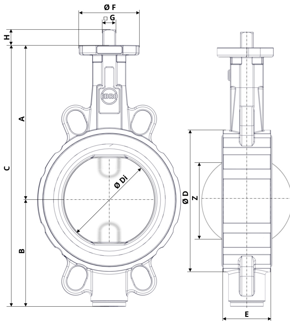
Fig. 3: Dimensiuni principale Z011-B
