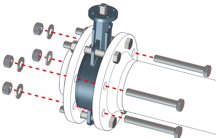
Fig. 9: Înșurubați clapeta interpusă între flanșe
