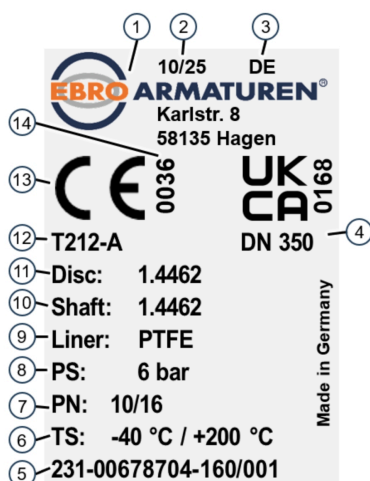
Fig. 1: Exemplo Placa de identificação
