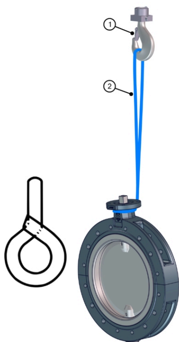
Fig. 6: Elevar a válvula de flange dupla com um guindaste
