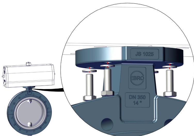
Fig. 7: Princípio Montagem dos componentes
