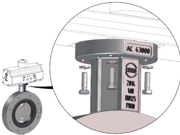
Fig. 7: Princípio Montagem dos componentes
