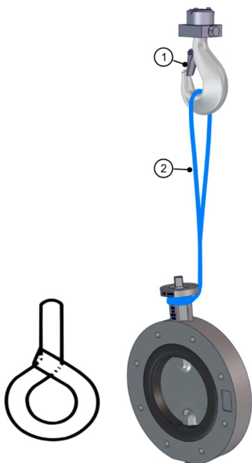
Fig. 6: Guindaste com válvula de flange completa
