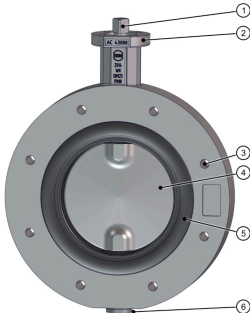
Fig. 2: Componentes
