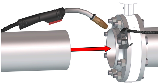
Fig. 10: Soldar o tubo com a flange
