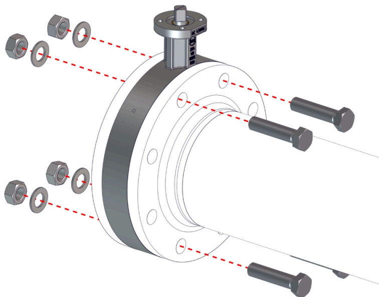
Fig. 8: Posicionar a válvula de flange integral
