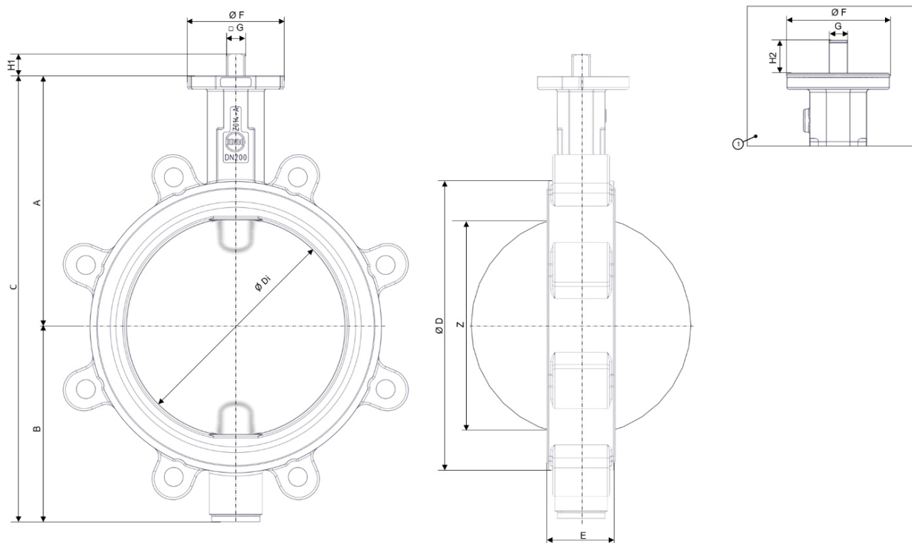
Fig. 3: Dimensões principais Z014-B
