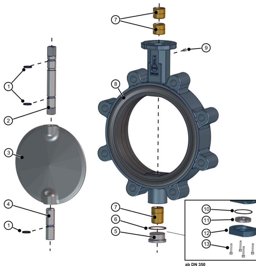
Fig. 15: Lista de peças Z014-B
