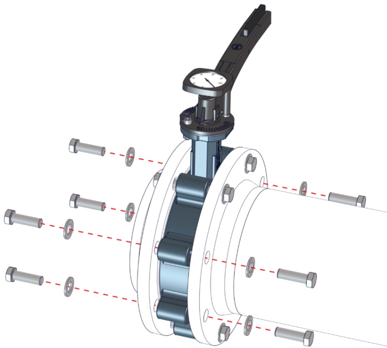
Fig. 9: Aparafusar a tampa da flange
