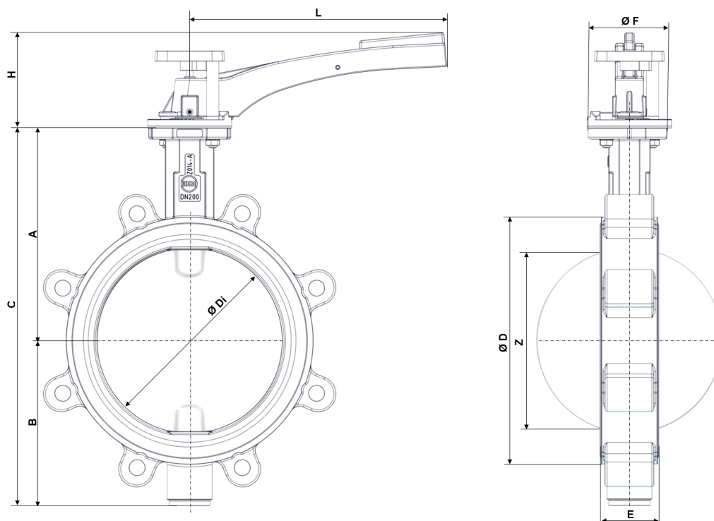
Fig. 3: Dimensões principais Z014-A THERM
