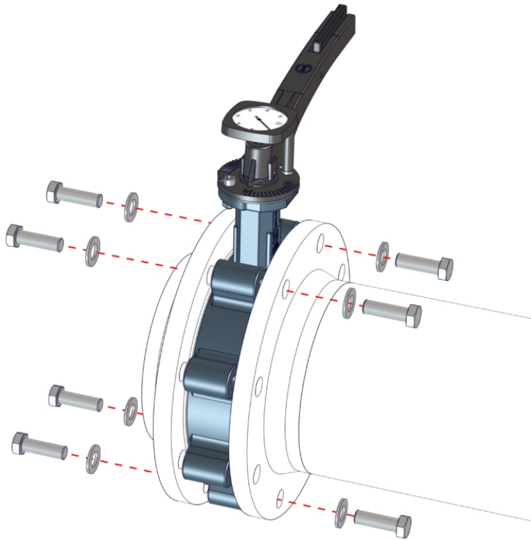
Fig. 8: Posicionar a válvula de flange
