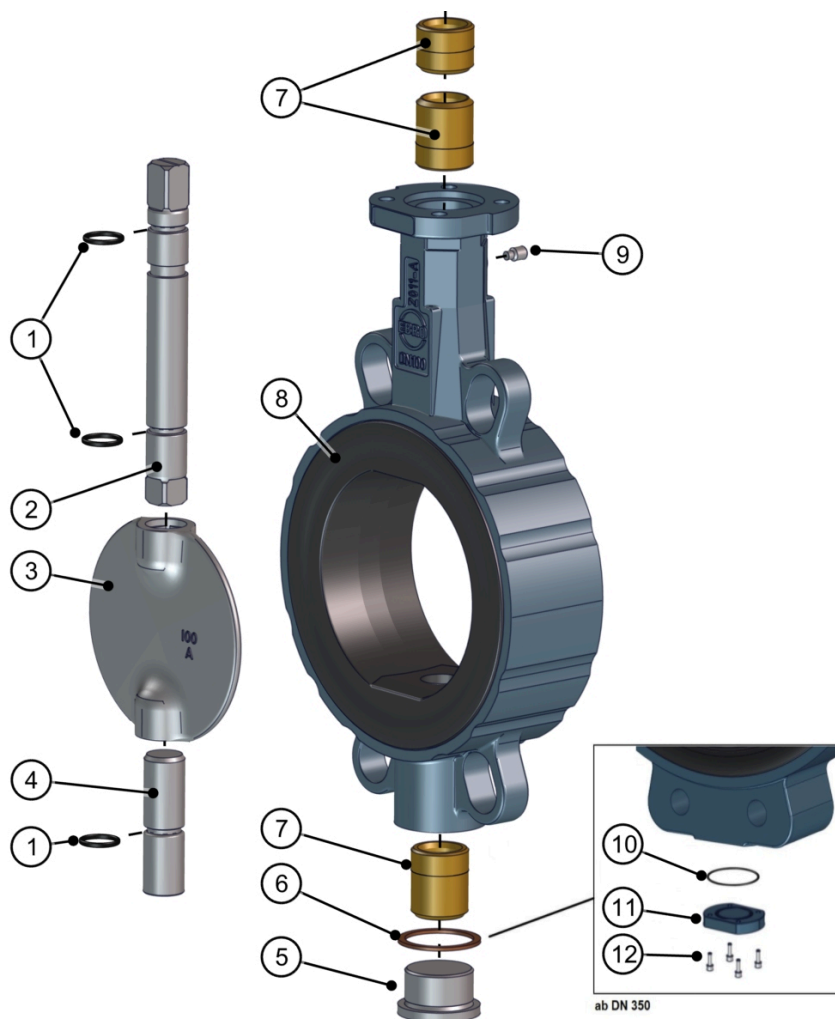
Fig. 15: Lista de peças Z011-B veio dividido
