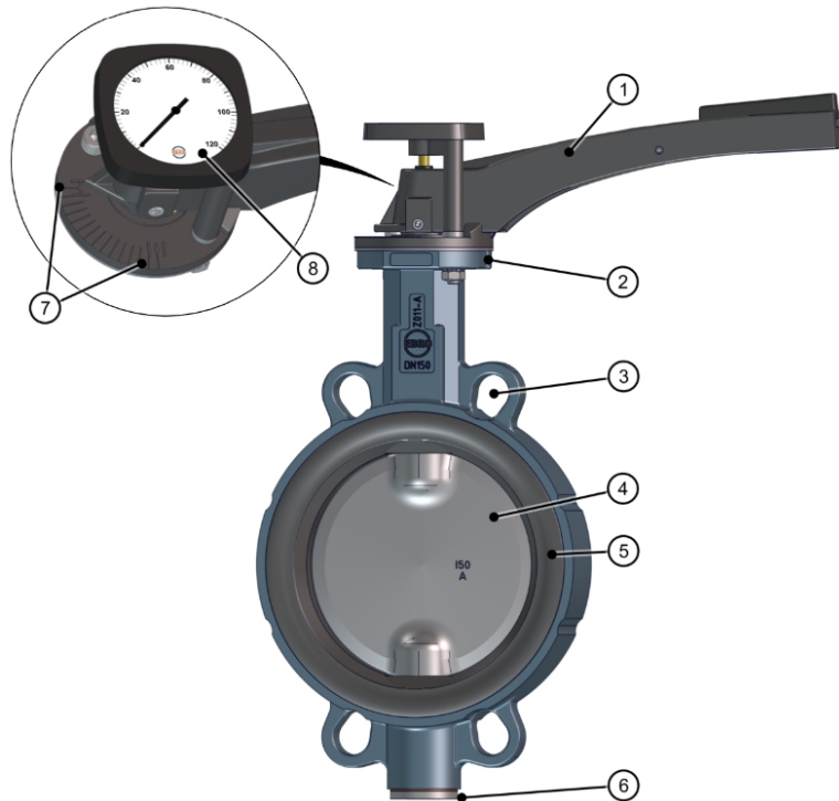
Fig. 2: Componentes
