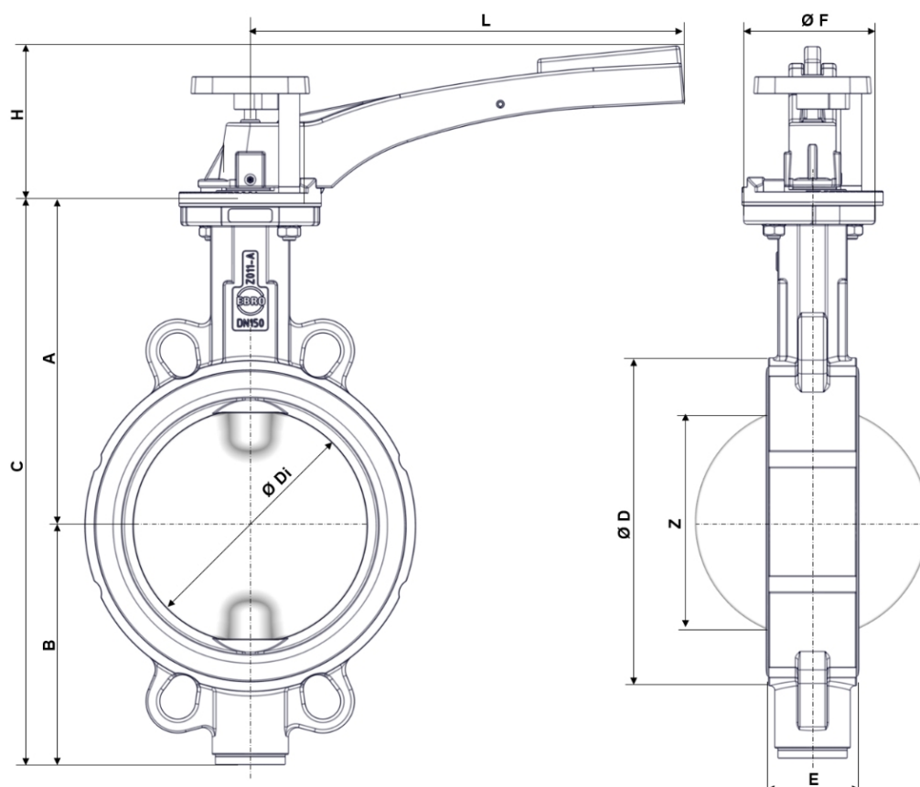
Fig. 3: Dimensões principais Z011-A THERM
