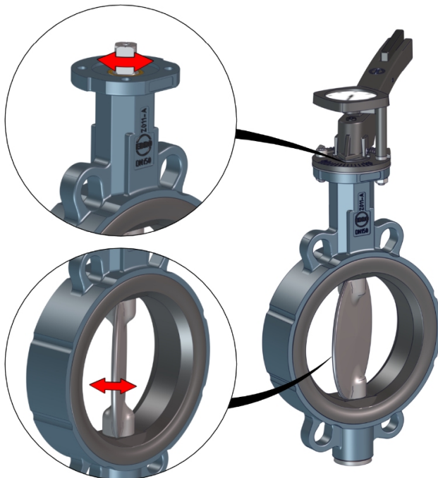
Fig. 4: Peças móveis
