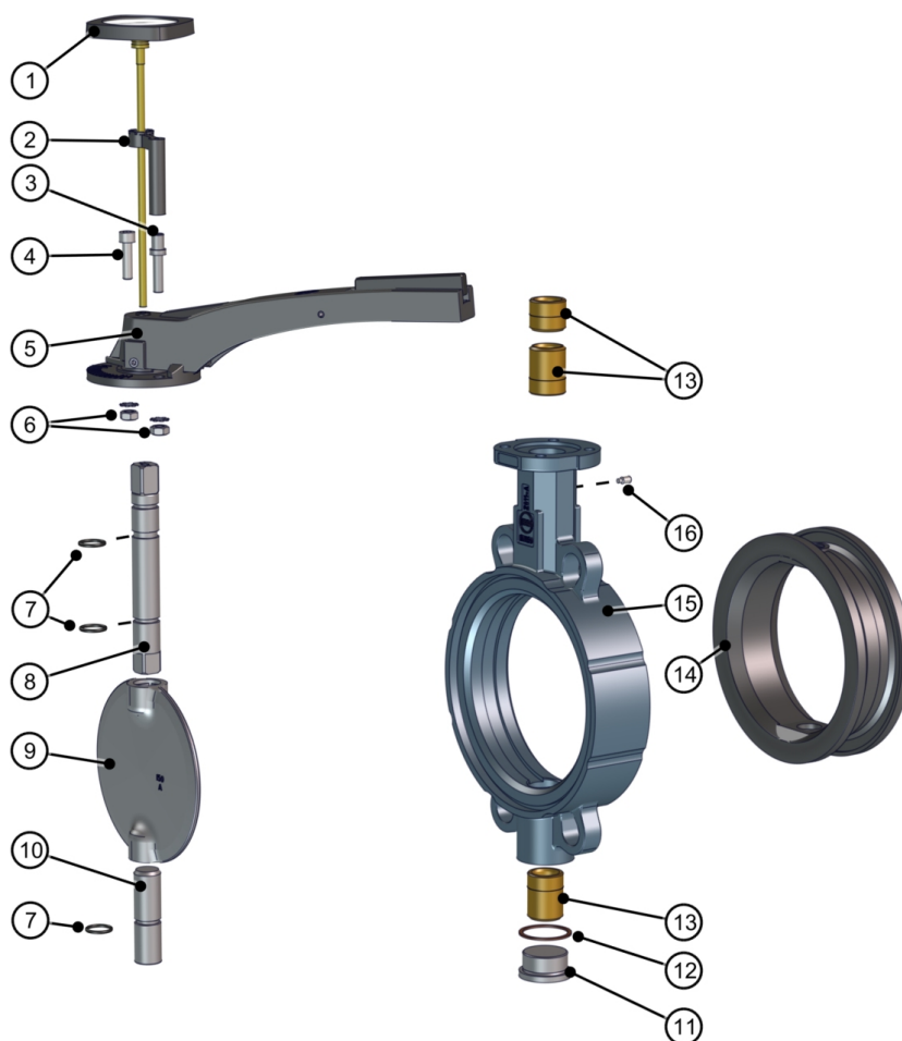
Fig. 16: Lista de peças Z011-A THERM
