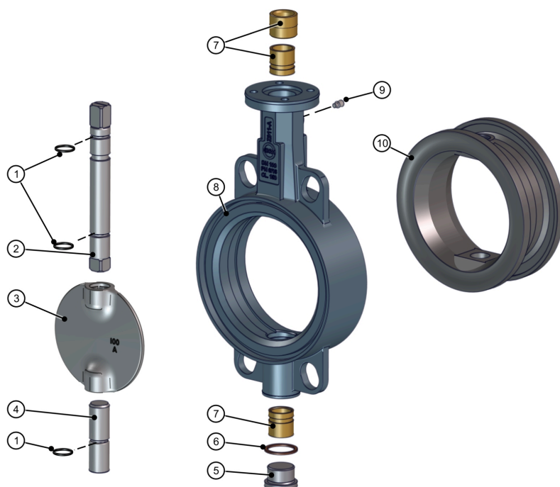
Fig. 15: Lista de peças Z011-AS
