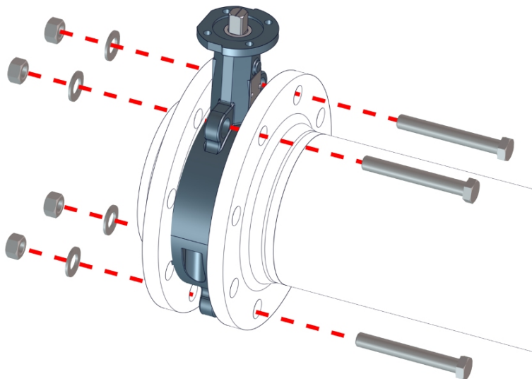
Rys. 8: Zwischenflanschklappe positionieren
