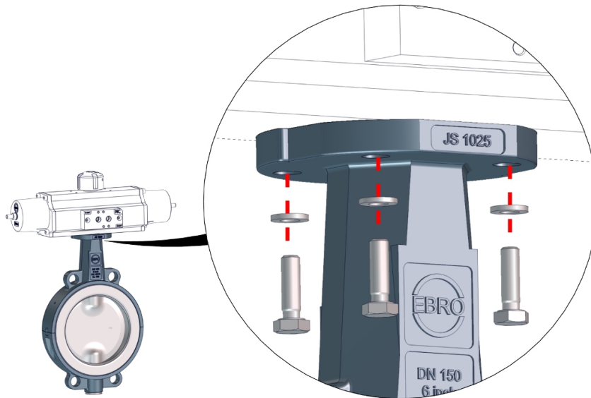
Rys. 7: Prinzip Komponenten montieren
