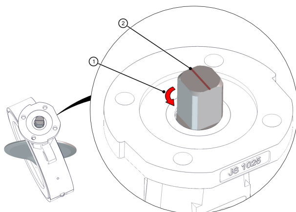
Rys. 14: Betätigungsrichtung
