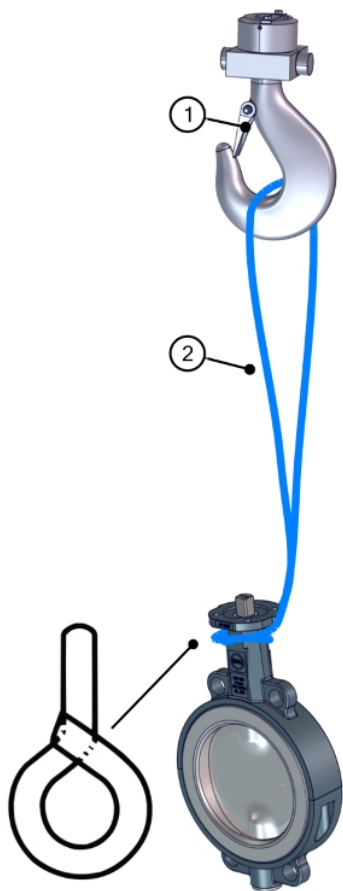
Rys. 6: Zwischenflanschklappe kranen
