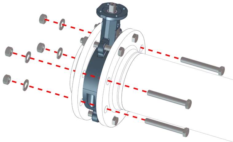
Rys. 9: Zwischenflanschklappe verschrauben
