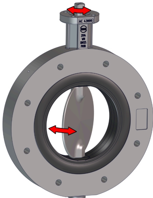
Rys. 4: Elementy ruchome
