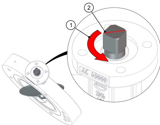
Rys. 14: Kierunek uruchomienia
