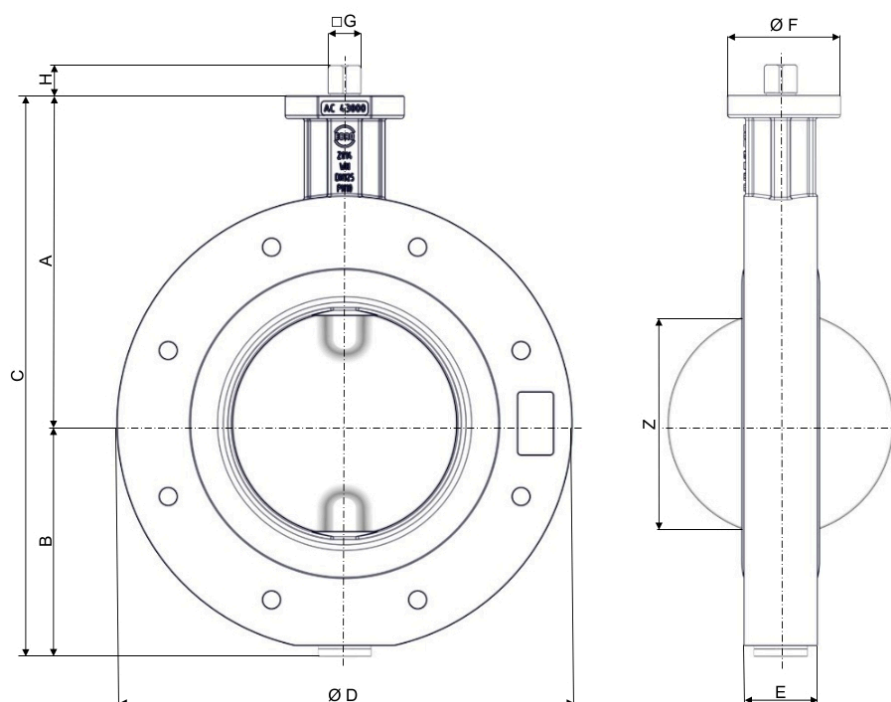
Rys. 3: Główne wymiary Z014-WN
