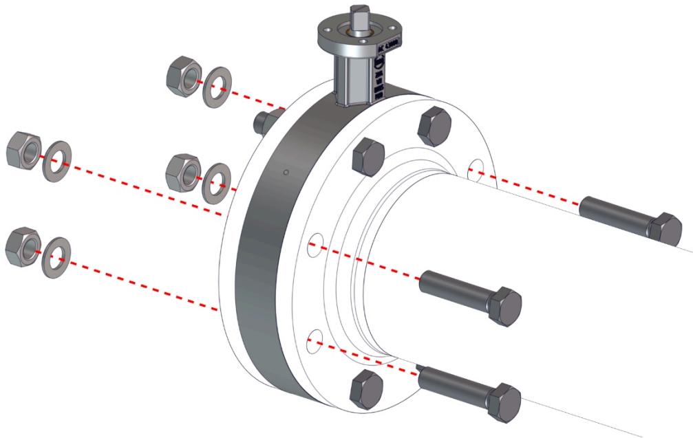
Rys. 9: Przykręcenie kłapy z pełnym kołnierzem
