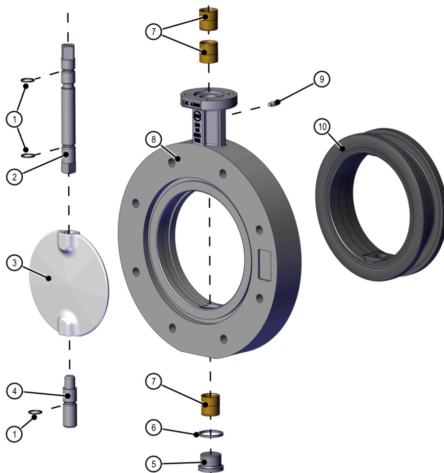
Rys. 15: Wykaz części Z014-WN
