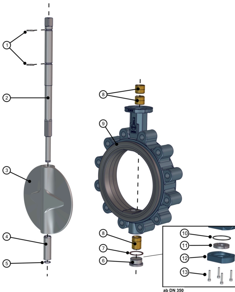
Rys. 16: Wykaz części wału TS 2014-B
