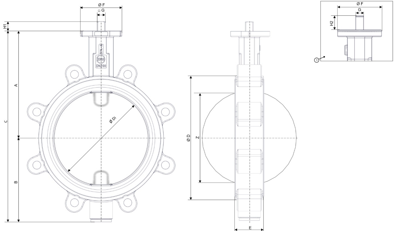
Rys. 3: Główne wymiary Z104-B
