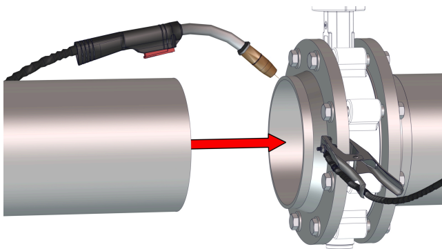
Rys. 10: Zespawanie rury z kołnierzem
