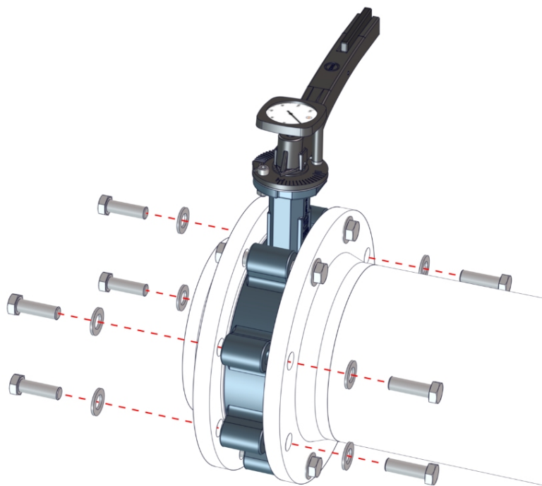
Rys. 9: Przykręcenie kłapy z kołnierzem przyłączeniowym
