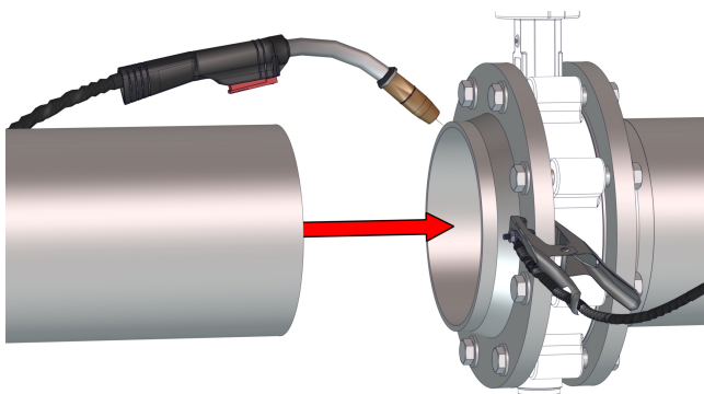
Rys. 10: Zespawanie rury z kołnierzem
