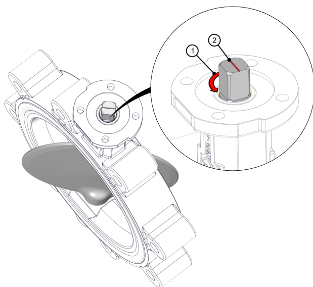
Rys. 14: Kierunek uruchomienia
