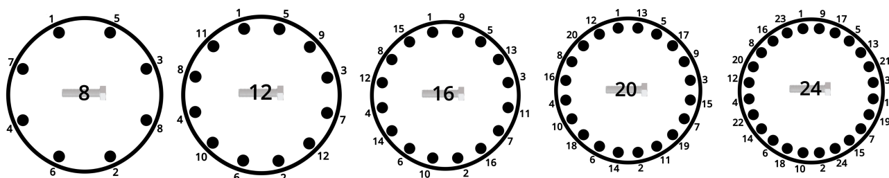
Rys. 12: Kolejność skręcania kołnierzowego złącza śrubowego rury
