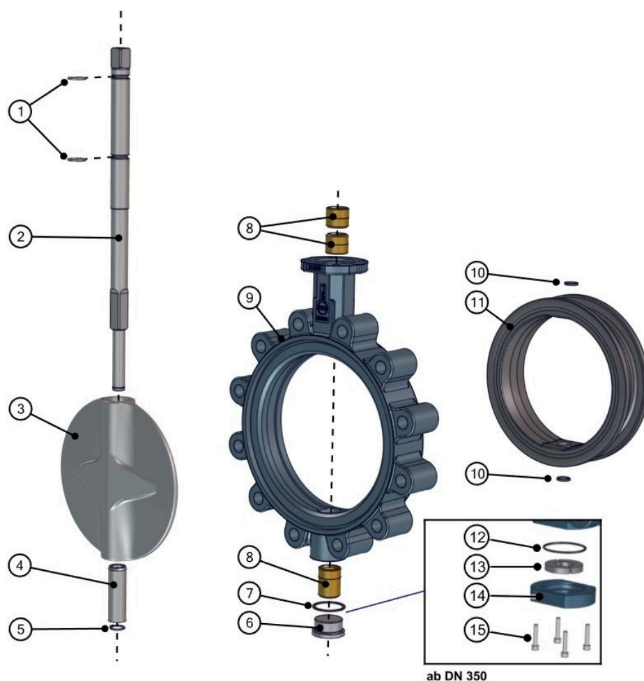
Rys. 16: Wykaz części wału TS Z014-A
