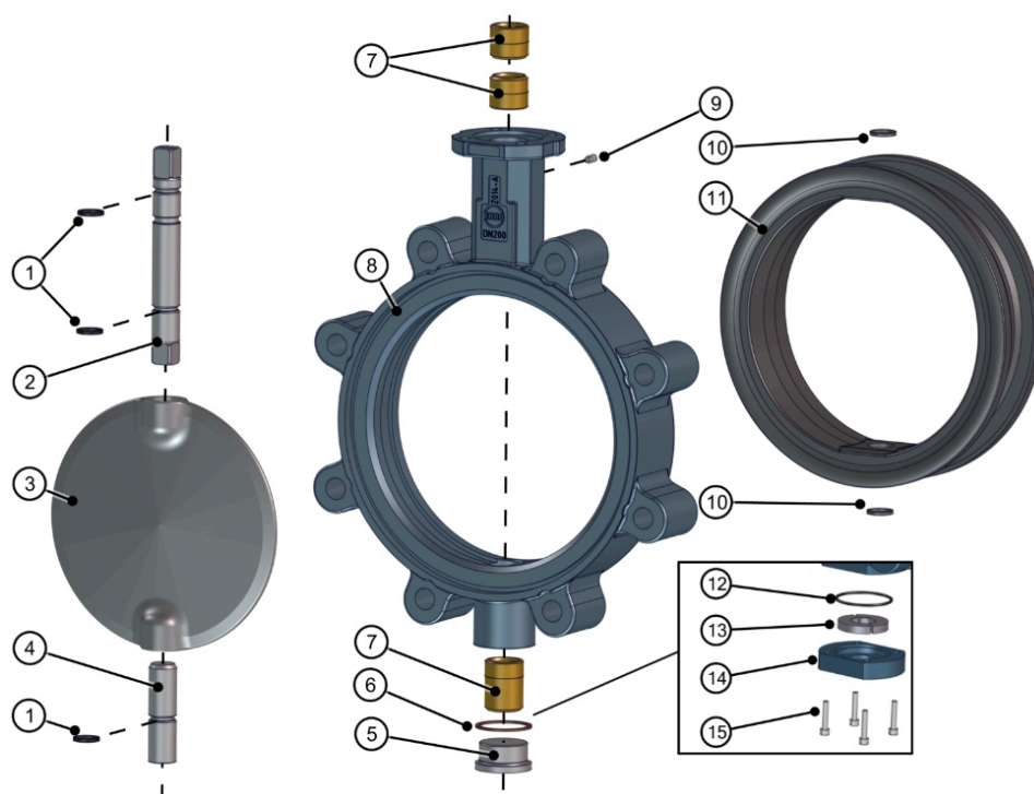
Rys. 15: Wykaz części Z014-A
