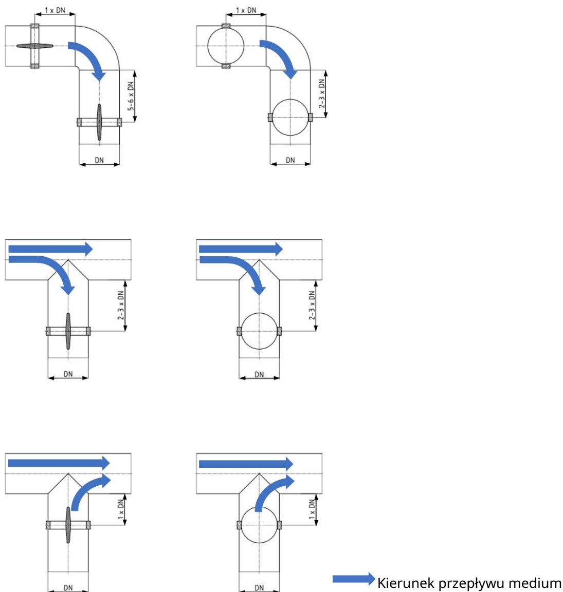
Rys. 11: Odstęp od odgałęzień rur
