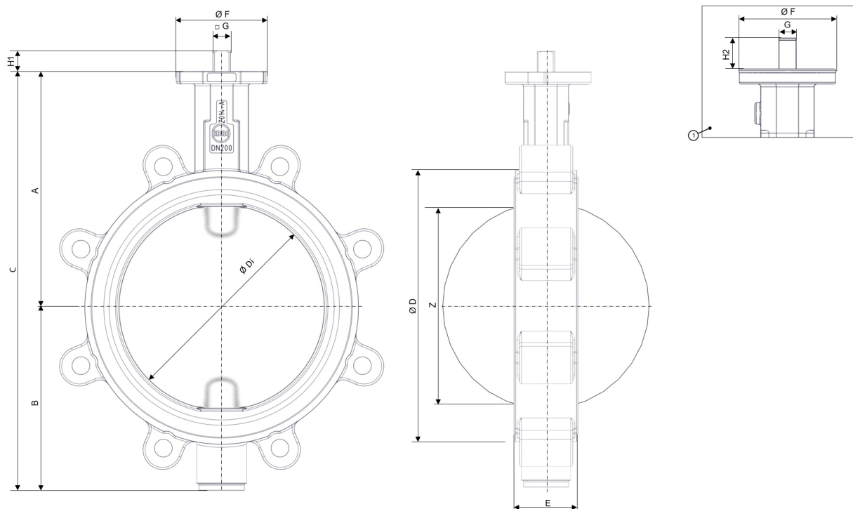
Rys. 3: Główne wymiary Z14-A
