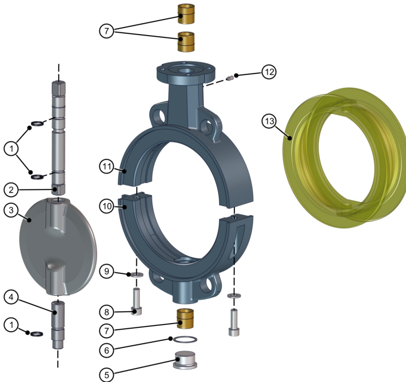
Rys. 15: Wykaz części Z011-GMX
