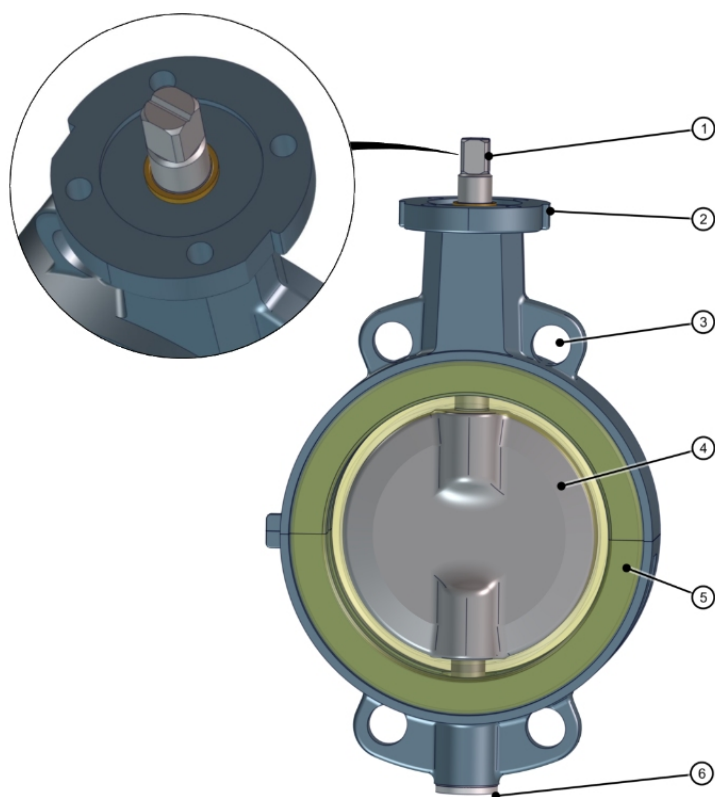
Rys. 2: Komponenty
