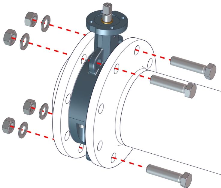
Rys. 8: Pozycjonowanie kłapy z kołnierzem pośrednim
