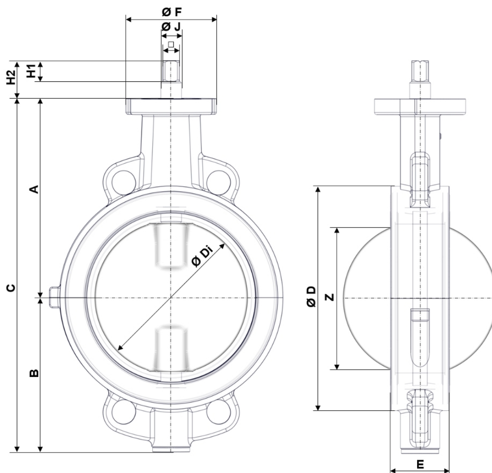
Rys. 3: Głównie wymiary Z011-GMX
