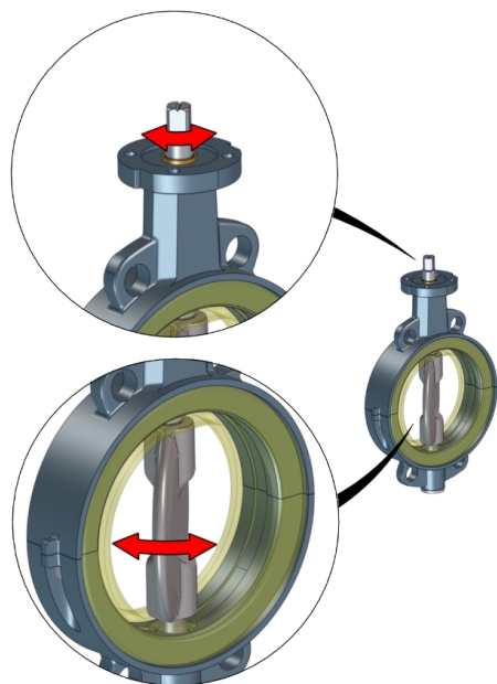
Rys. 4: Elementy ruchome
