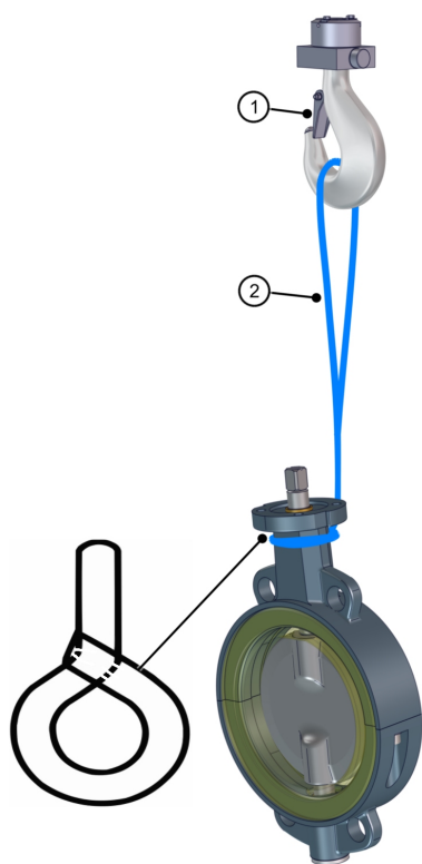
Rys. 6: Przenoszenie kłapy z kołnierzem pośrednim przy użyciu dźwigu
