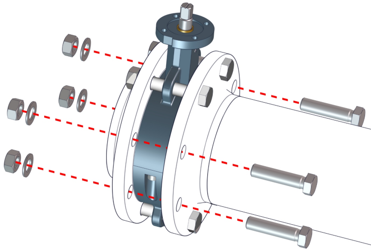
Rys. 9: Przykręcenie klapy z kołnierzem pośrednim
