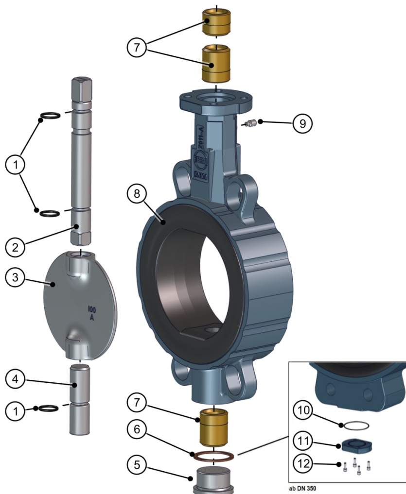
Rys. 15: Wykaz części wału podzielonego Z011
