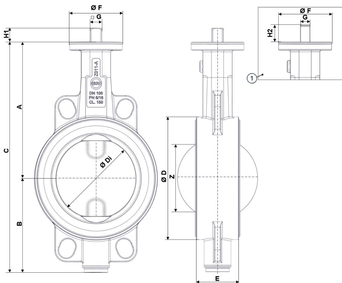
Rys. 3: Główne wymiary Z011-AS
