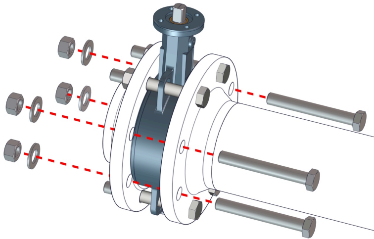
Rys. 9: Przykręcenie kłapy z kołnierzem pośrednim
