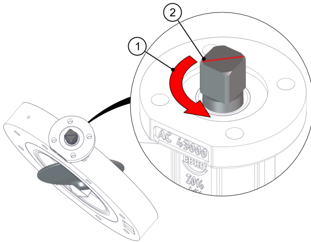
Fig. 14: Aktiveringsretning
