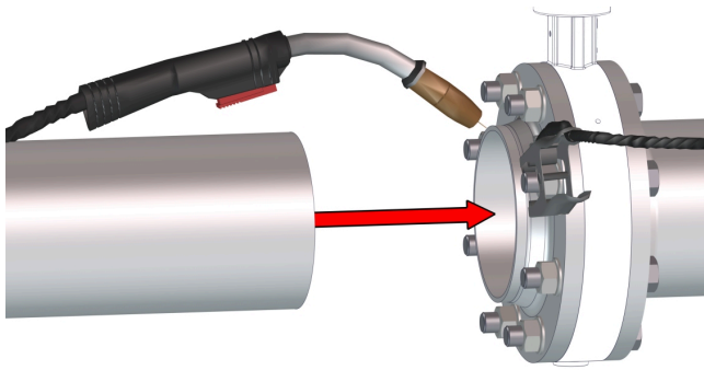
Fig. 10: Sveise røret med flens
