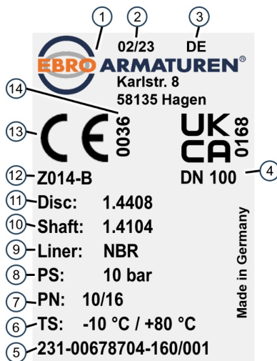
Fig. 1: Eksempel på typeskilt
