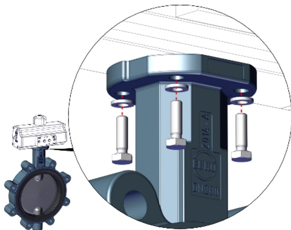
Fig. 7: Prinsipp for montering av komponentene
