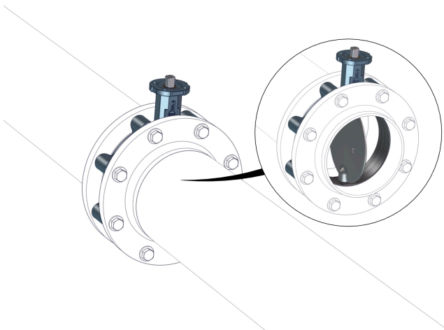
Fig. 13: Skyll røret
