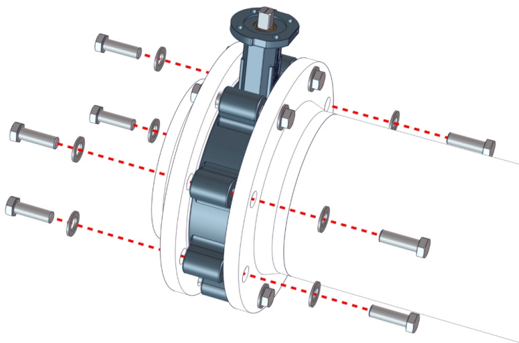
Fig. 9: Skru fast flensspjeldet
