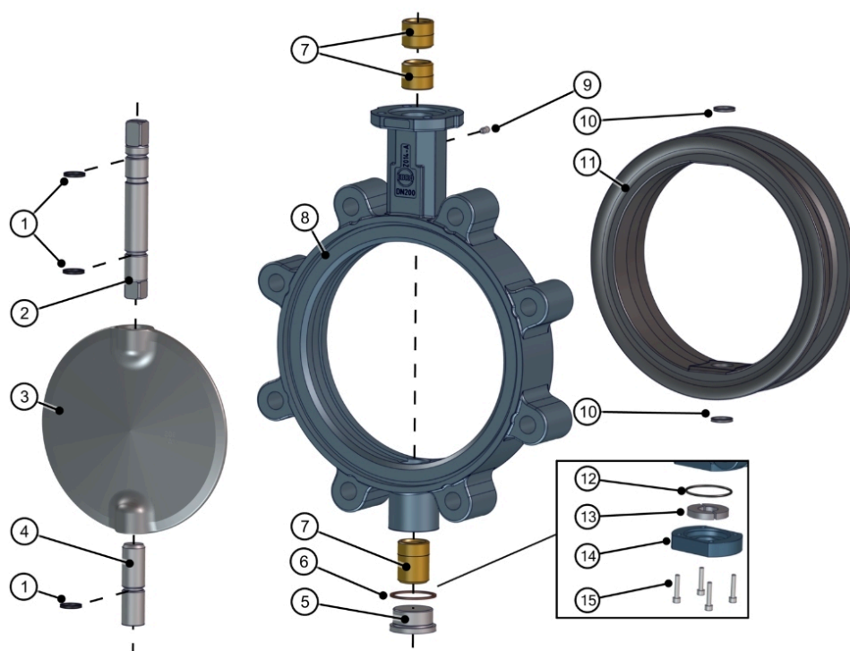
Fig. 15: Stykkliste Z014-A
