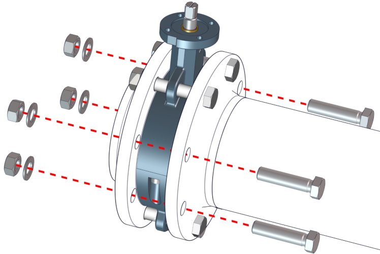
Fig. 9: Skru fast mellomflensspjeldet
