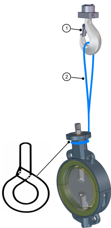
Fig. 6: Bruk kran på mellomflensspjeldet
