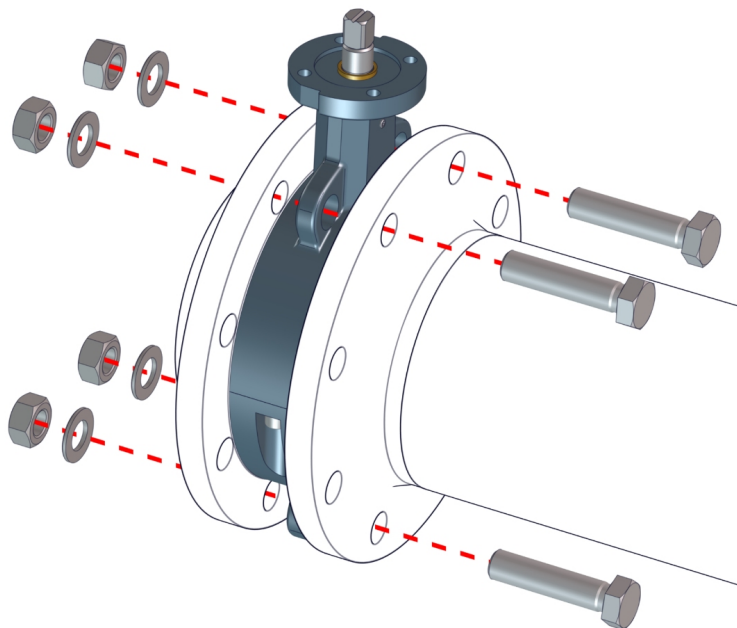
Fig. 8: Posisjonere mellomflensspjeld
