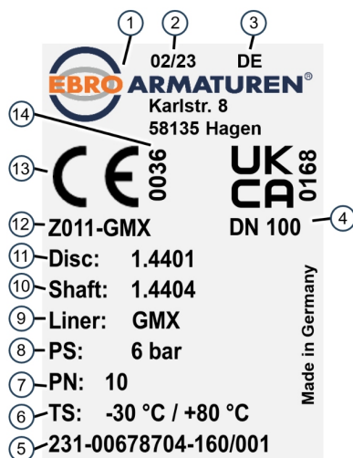
Fig. 1: Eksempel på typeskilt
