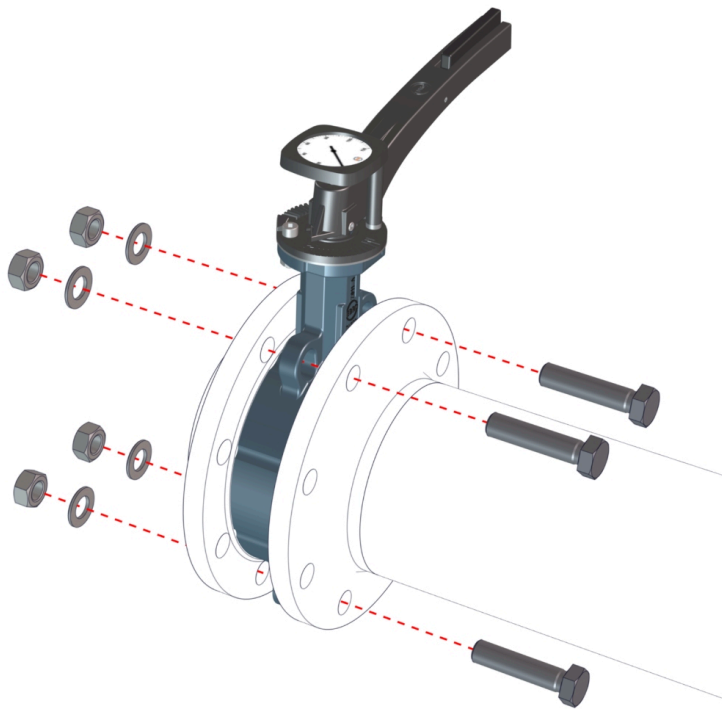
Fig. 8: Posisjonere mellomflensspjeld
