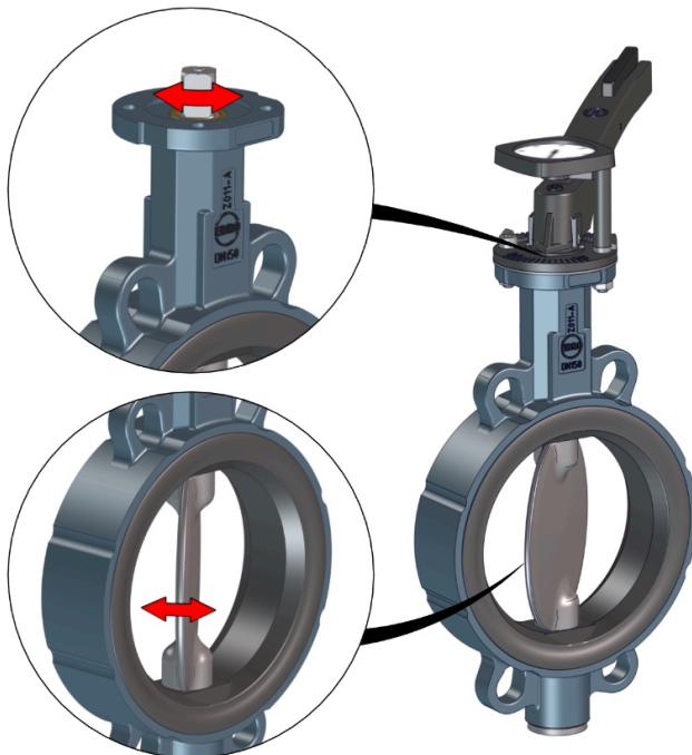
Fig. 4: Bevegelige deler
