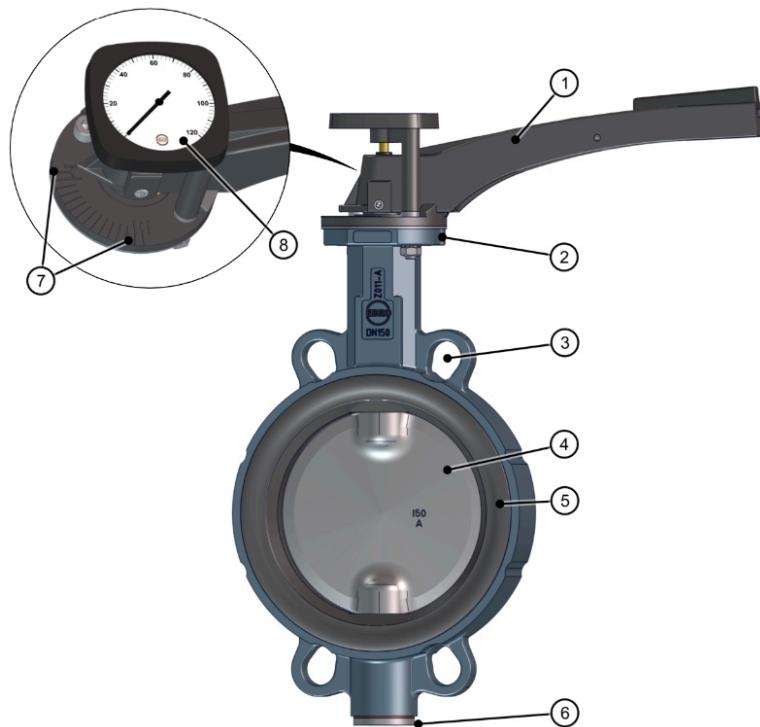
Fig. 2: Komponenter
