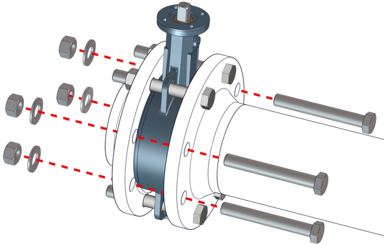
Fig. 9: Skru fast mellomflensspjeldet
