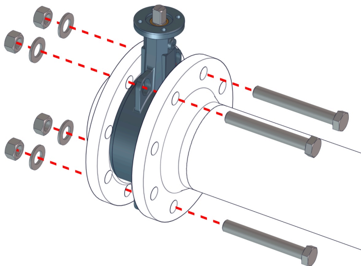
Fig. 8: Posisjonere mellomflensspjeld
