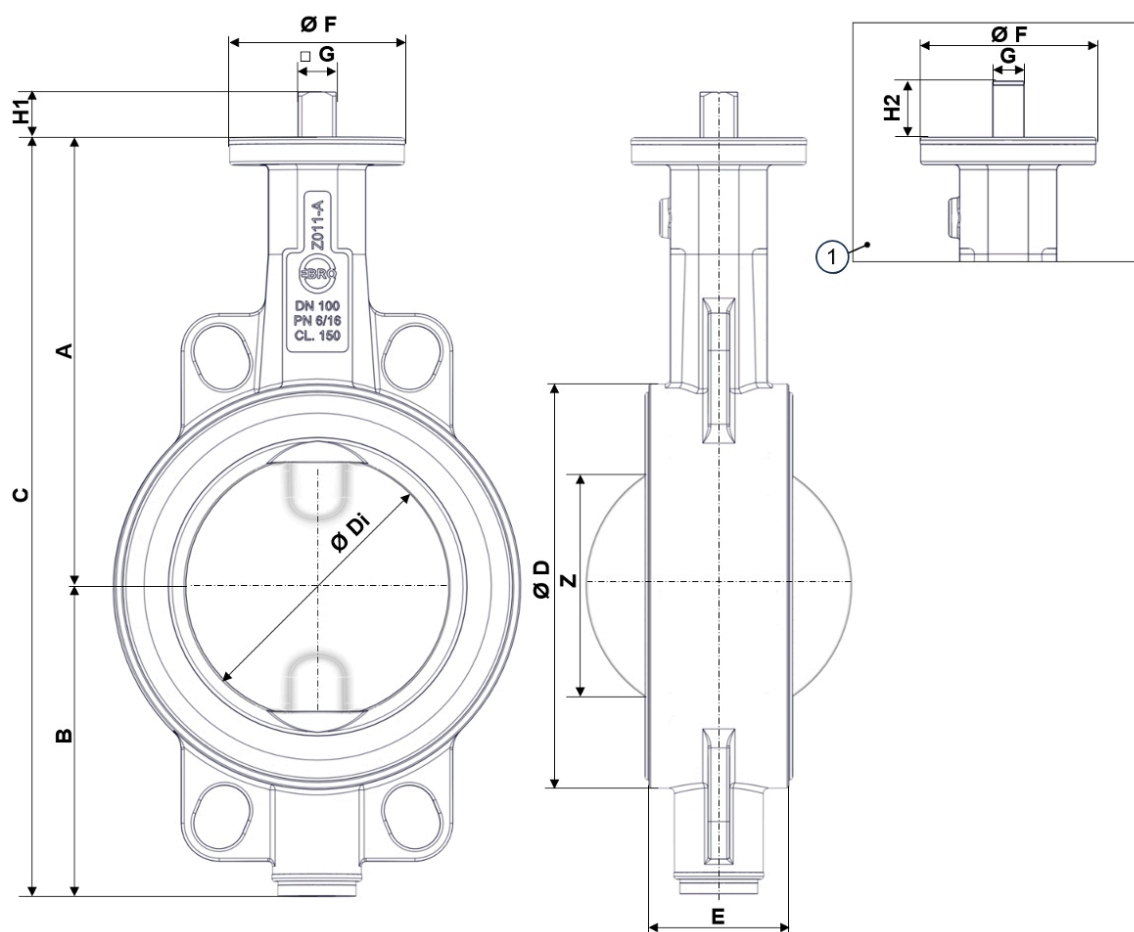
Fig. 3: Hovedmål Z011-AS
