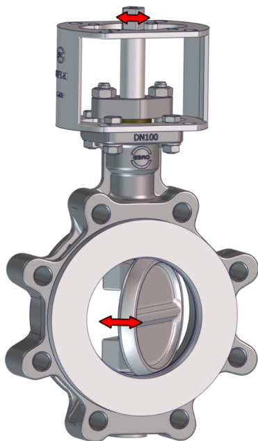
Att. 4: Kustīgās daļas
