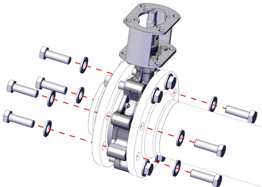
Att. 9: Flanča tauriņvārsta uzskrūvēšana
