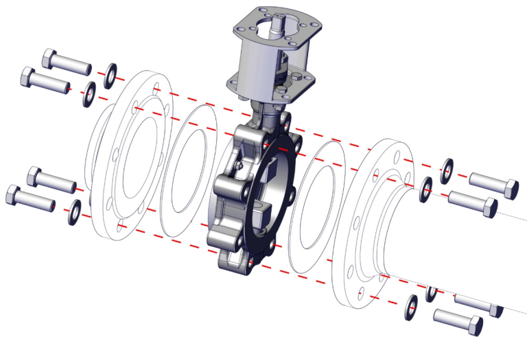
Att. 8: Flanča tauriņvārsta pozicionēšana
