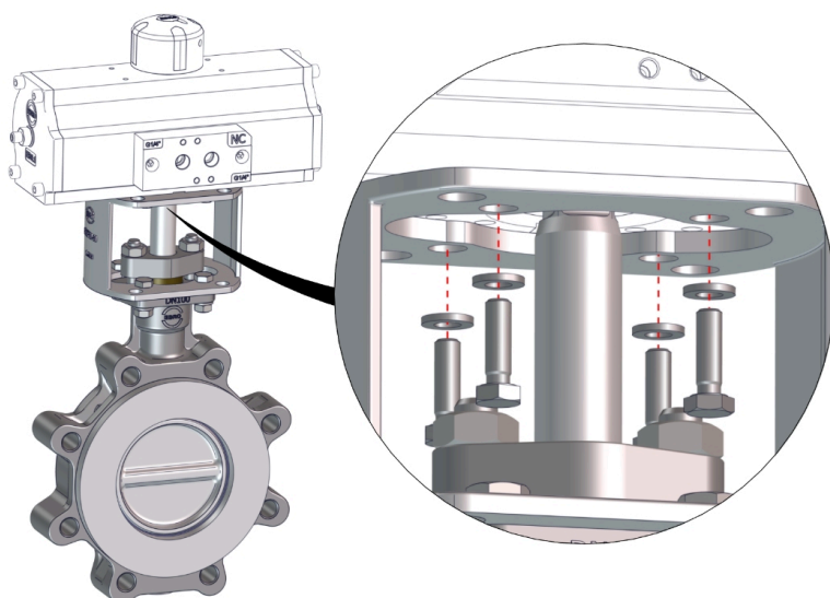
Att. 7: Komponentu montāžas princips
