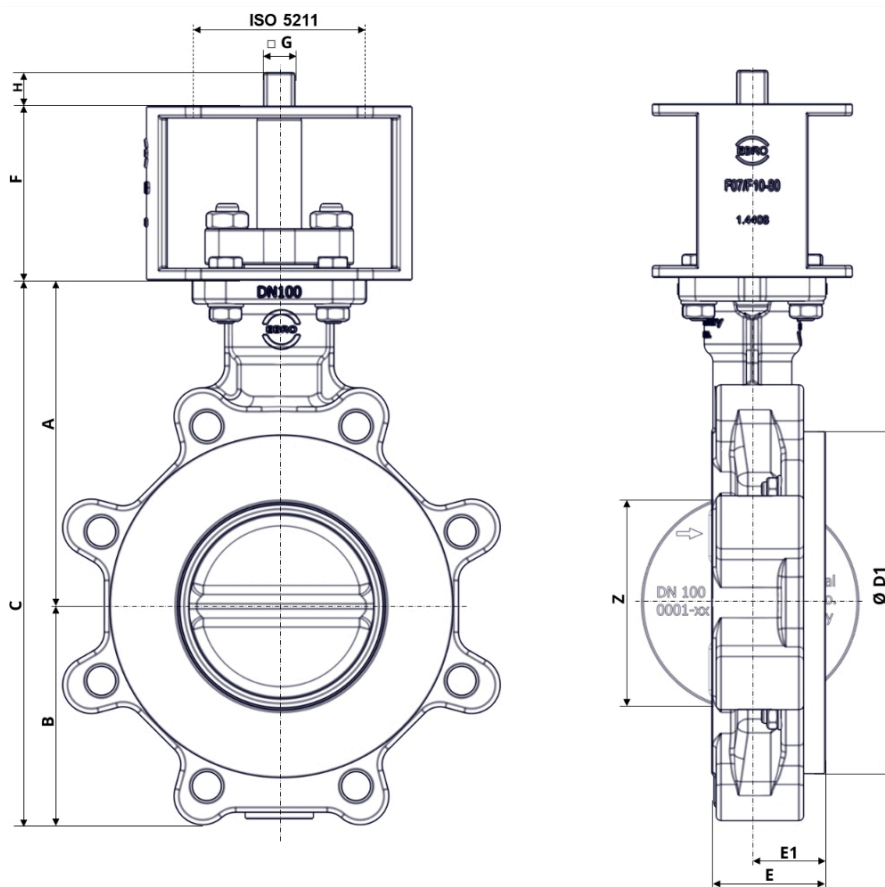
Att. 3: Galvenie izmēri HP114-HF
