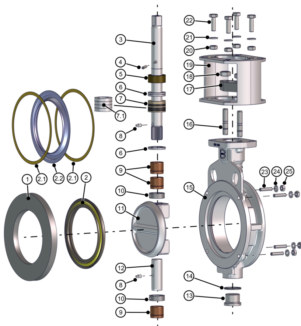
Att. 15: Detaļu saraksts HP111-HF
