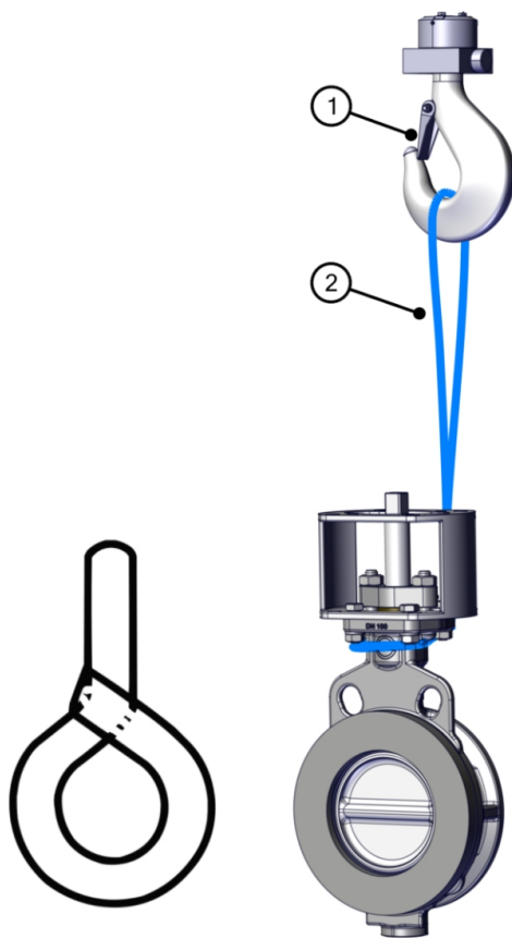
Att. 6: Starpflaņa tauriņvārsta pacelšana
