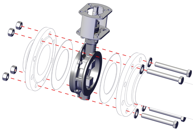
Att. 8: Starpflaņa tauriņvārsta pozicionēšana
