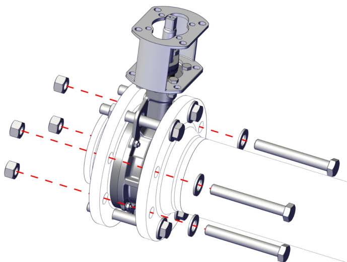
Att. 9: Starpposma flanča tauriņvārsta uzskrūvēšana
