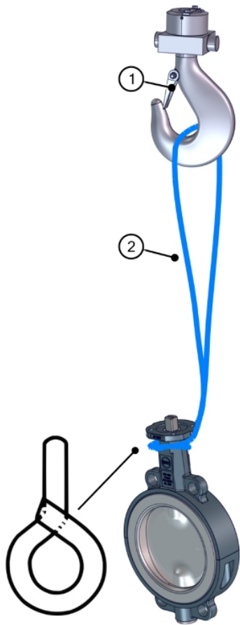
Att. 6: Zwischenflanschklappe kranen
