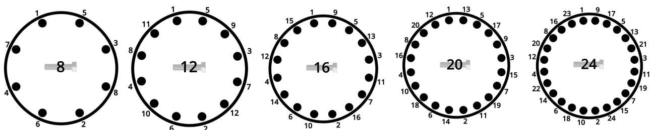
Att. 12: Cauruļvada atloka skrūvju pievilšanas secība
