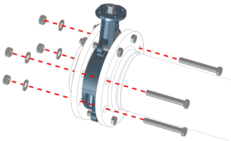
Att. 9: Zwischenflanschklappe verschrauben
