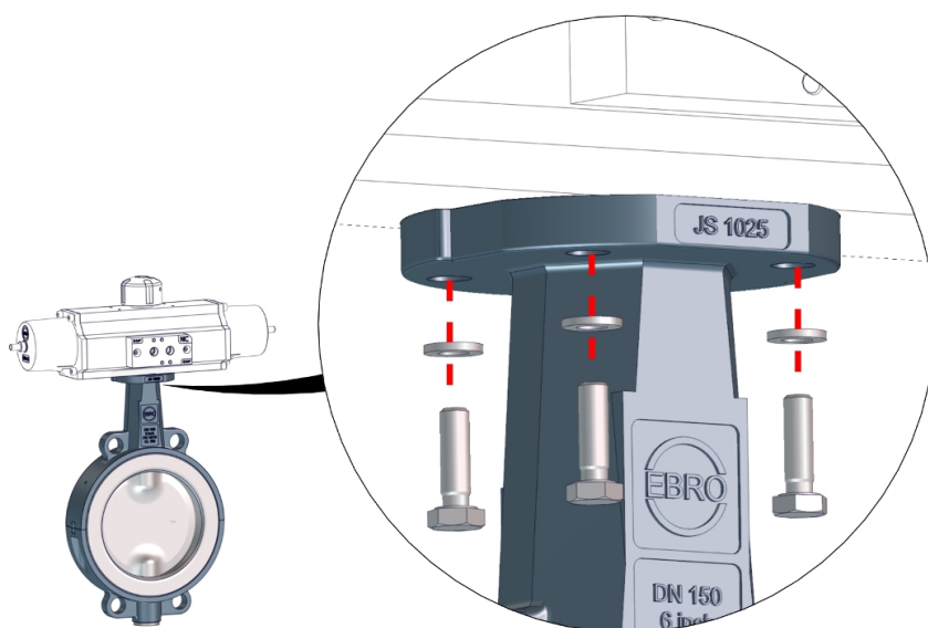
Att. 7: Prinzip Komponenten montieren
