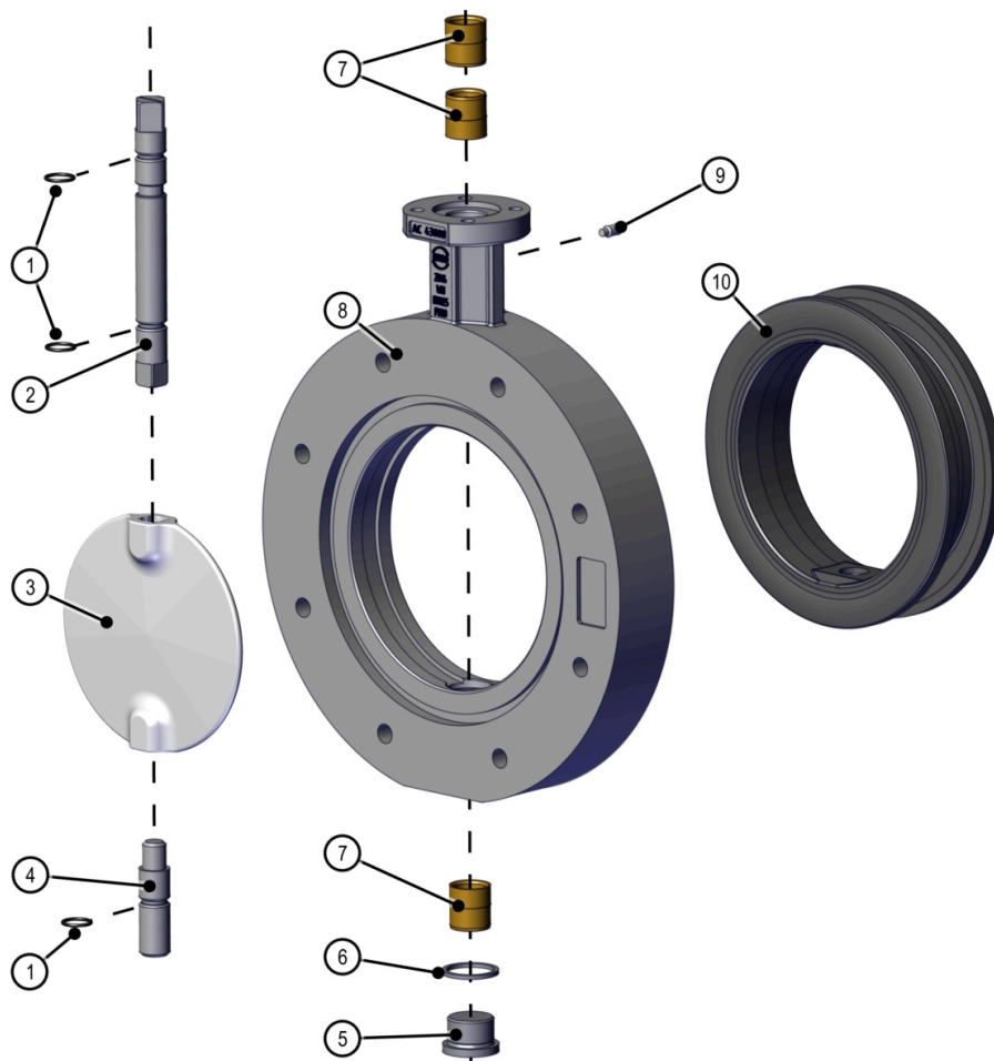
Att. 15: Detaļu saraksts Z014-WN
