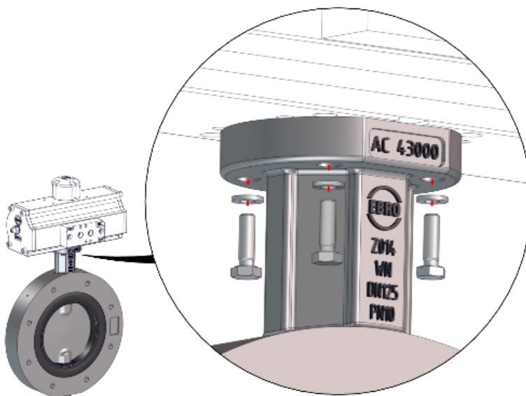
Att. 7: Komponentu montāžas princips
