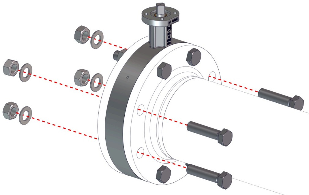
Att. 9: Pilna flanča tauriņvārsta uzskrūvēšana
