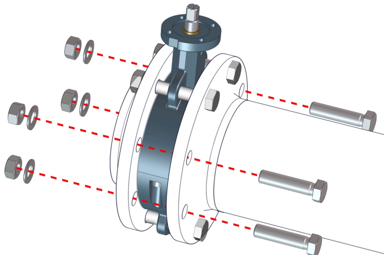
Att. 9: Starpflaņa tauriņvārsta uzskrūvēšana
