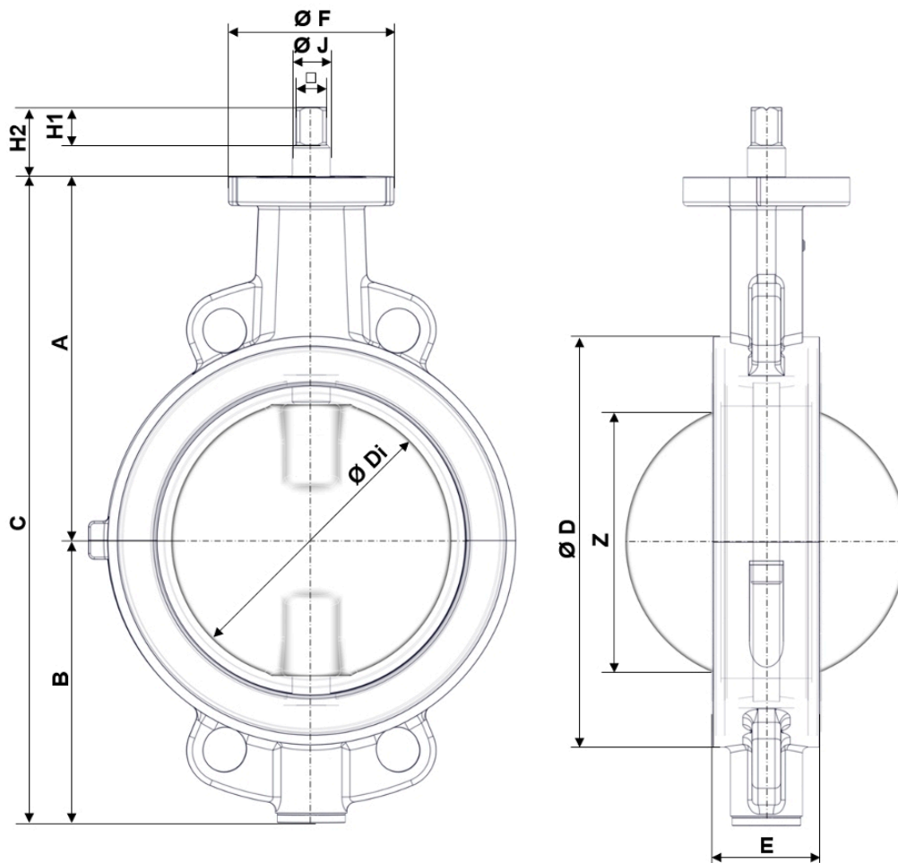
Att. 3: Galvenie izmēri Z011-GMX
