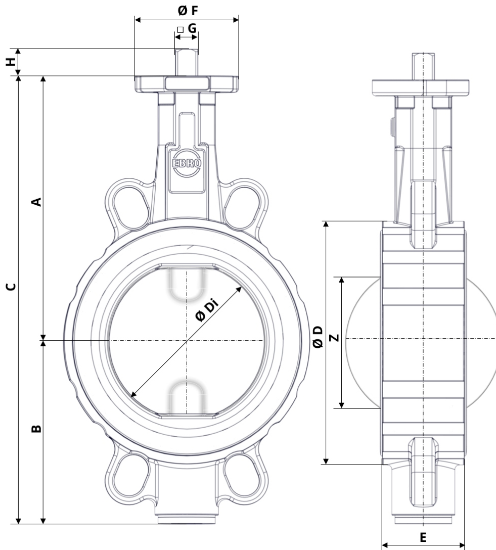
Att. 3: Galvenie izmēri Z011-B
