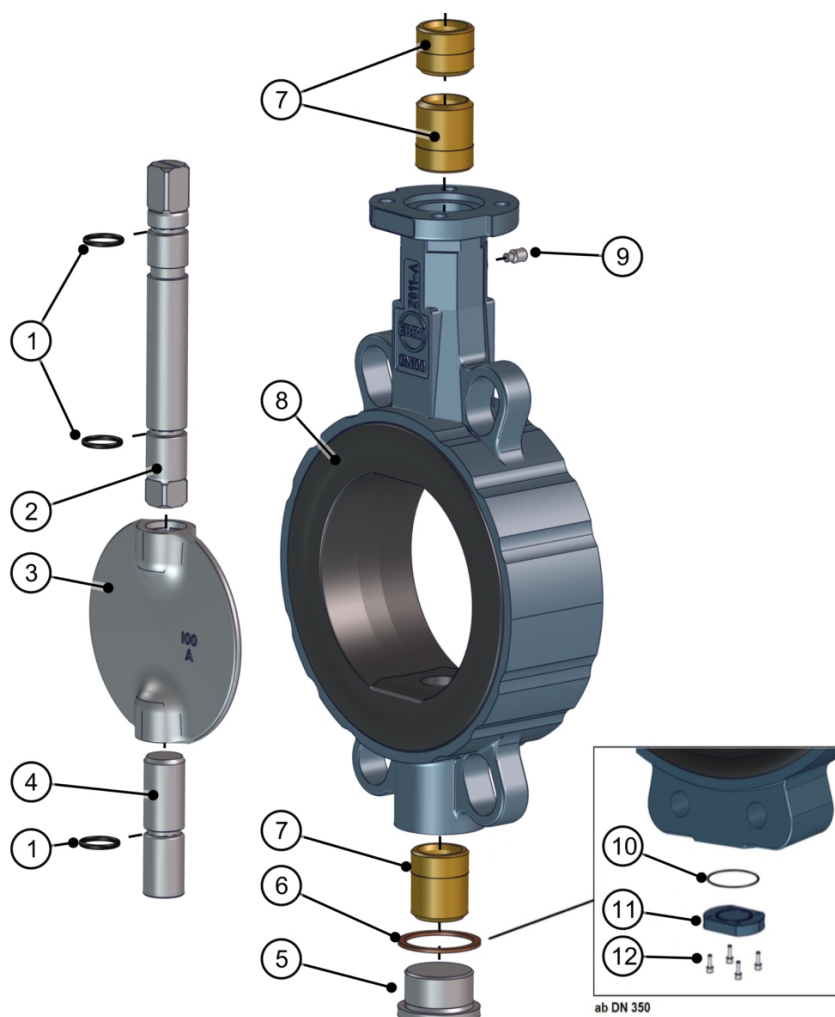
Att. 15: Materiālu saraksts Z011-B dalītā vārpsta
