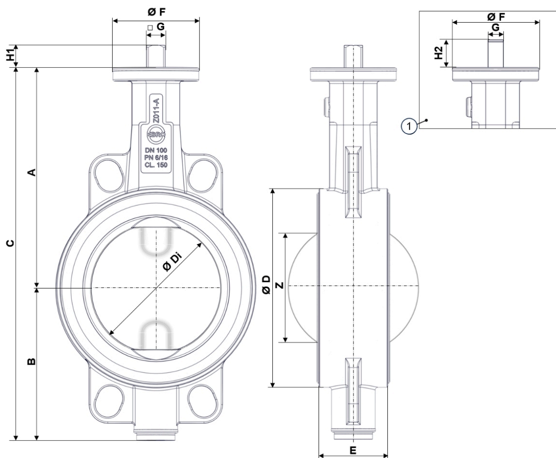
Att. 3: Galvenie izmēri Z011-AS
