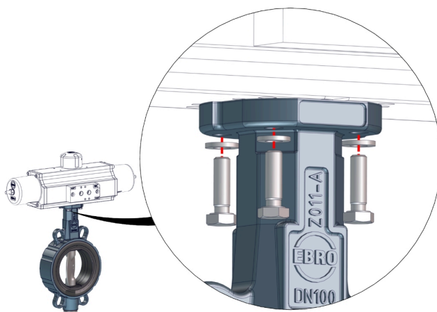
Att. 7: Komponentu montāžas princips
