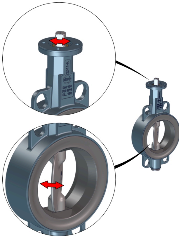
Att. 4: Kustīgās daļas
