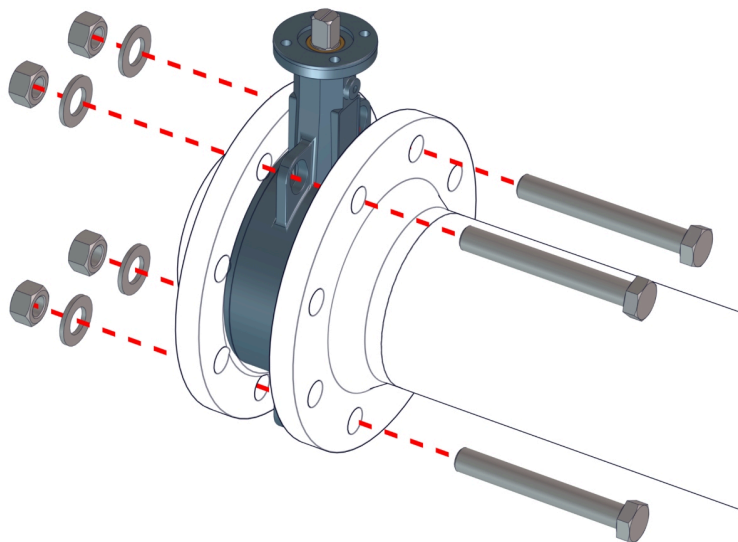
Att. 8: Starpflaņa tauriņvārsta pozicionēšana
