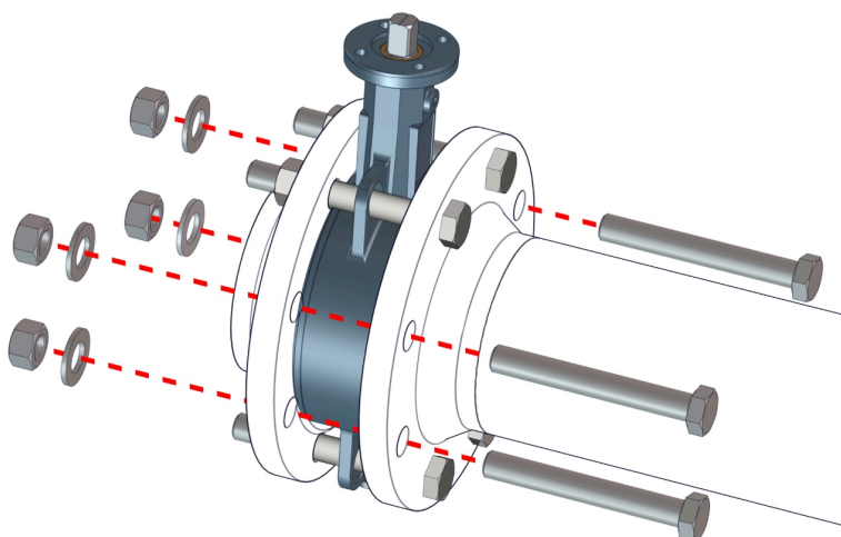
Att. 9: Starpflaņa tauriņvārsta uzskrūvēšana
