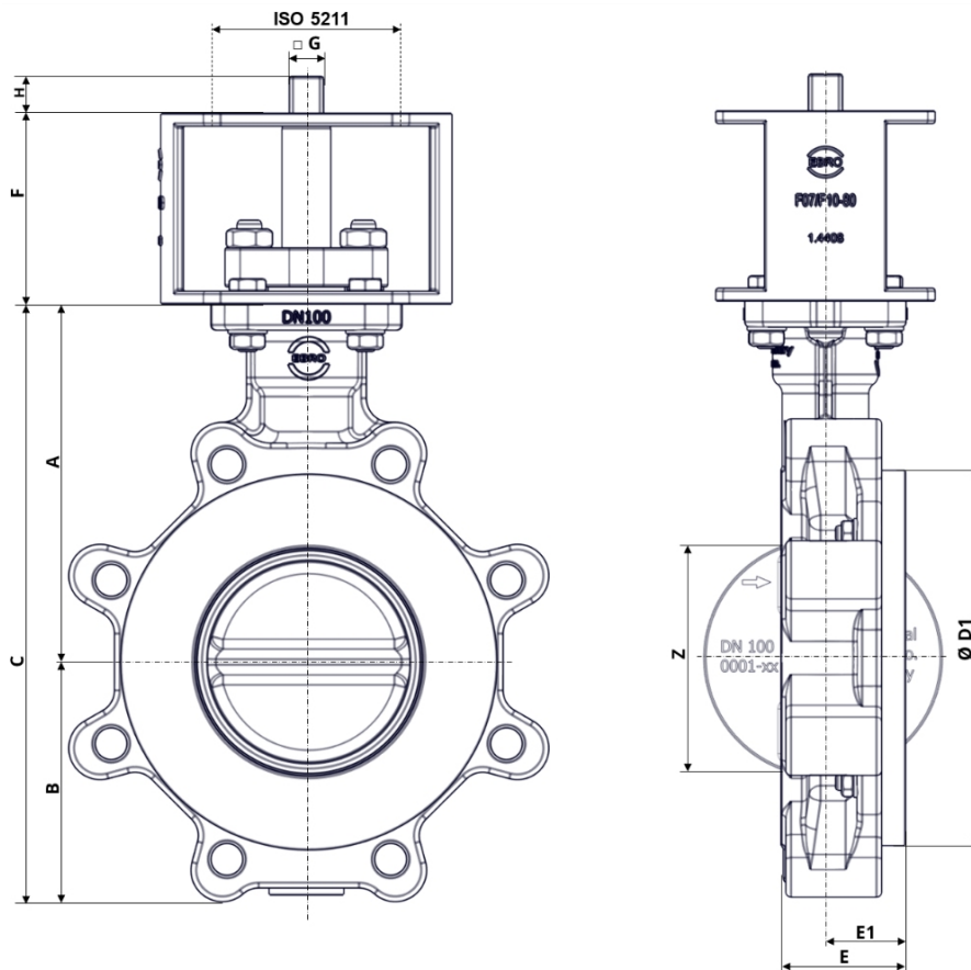
Paf. 3: HP114-HF pagrindiniai matmenys
