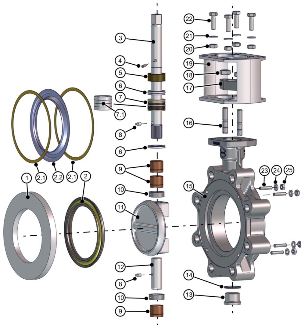
Paf. 15: HP114-HF dalių sąrašas
