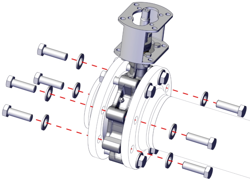
Paf. 9: Sparninio vožtuvo su iškyšomis prisukimas
