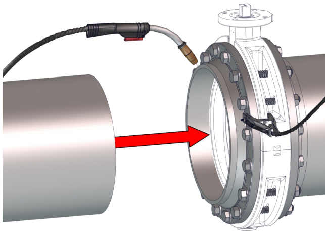
Paf. 10: Vamzdžio ir jungės suvirinimas
