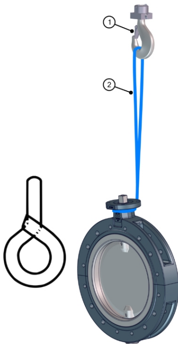
Paf. 6: Sklendės su dviguba jungė prikabinimas prie krano
