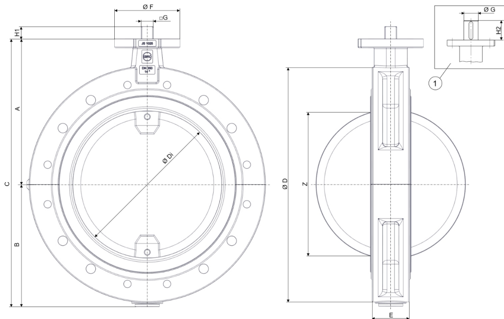
Paf. 3: T212-A pagrindiniai matmenys
