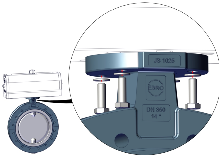
Paf. 7: Komponentų montavimo principas
