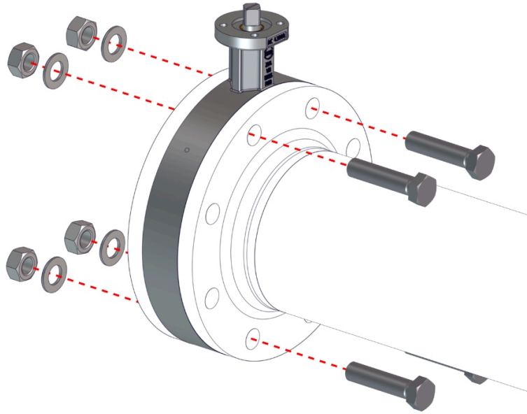
Paf. 8: Priglundančio sparninio vožtuvo padėties nustatymas
