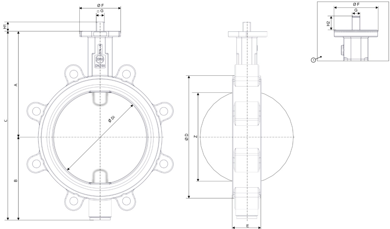
Paf. 3: Z014-B pagrindiniai matmenys
