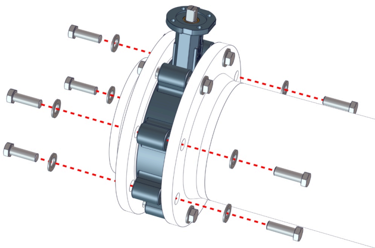
Paf. 9: Sparinio vožtuvo su iškyšomis prisukimas
