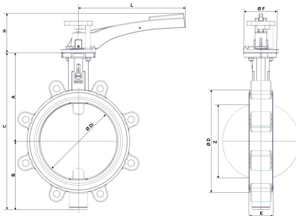
Paf. 3: Z014-A THERM pagrindiniai matmenys
