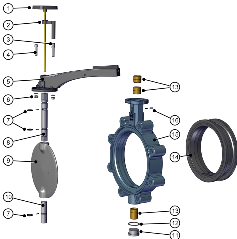
Paf. 16: Z014-A THERM dalių sąrašas
