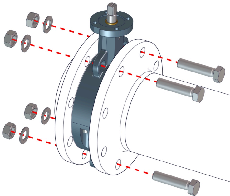
Paf. 8: Tarpjunginio sparninio vožtuvo padėties nustatymas
