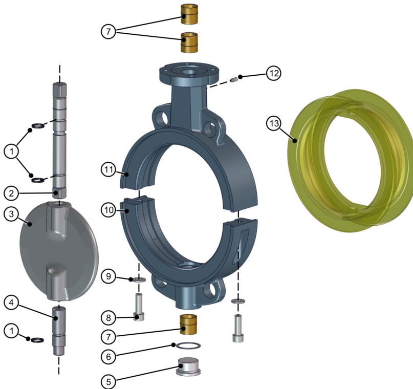
Paf. 15: Dalių sąrašas Z011-GMX
