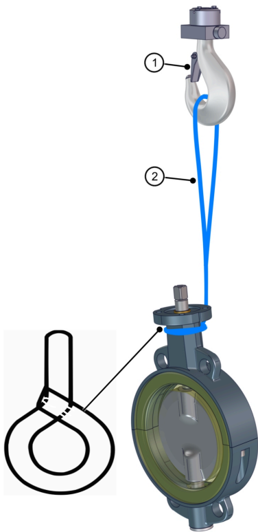
Paf. 6: Tarpjunginio sparninio vožtuvo prikabinimas prie krano
