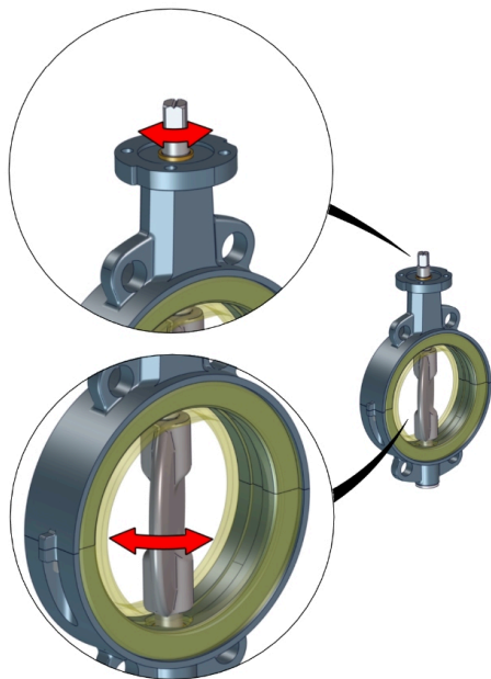
Paf. 4: Judančios dalys
