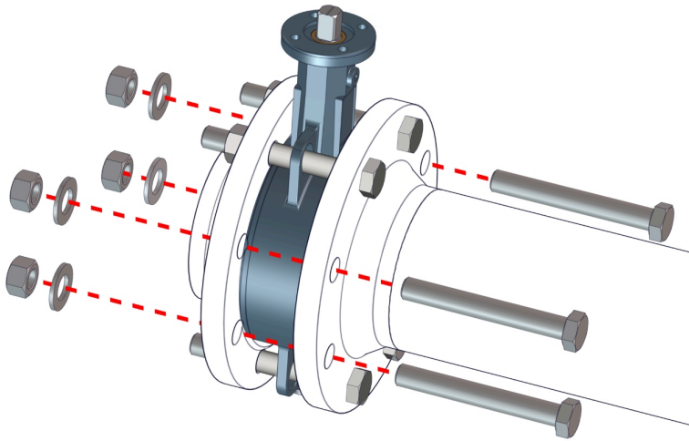
Paf. 9: Tarpjunginio sparninio vožtuvo prisukimas
