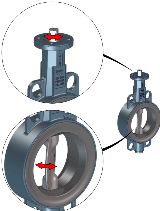
Paf. 4: Judančios dalys
