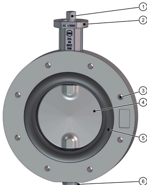
Fig. 2: Componenti
