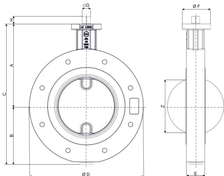
Fig. 3: Dimensioni principali Z014-WN
