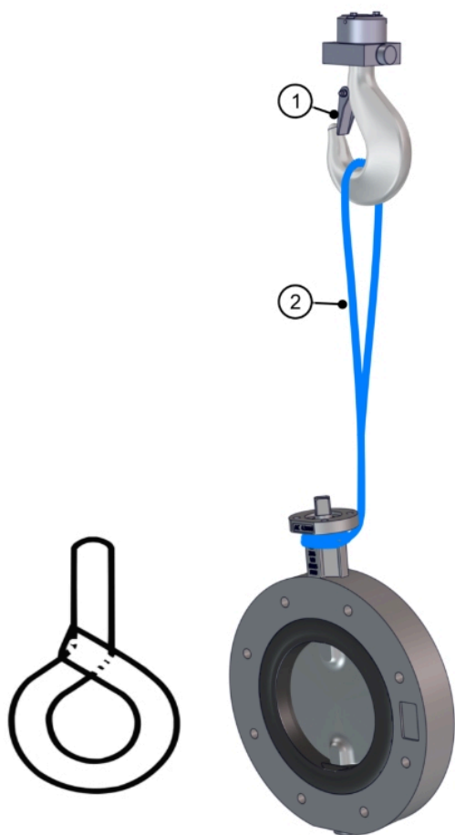
Fig. 6: Trasporto valvola a farfalla a flangia piena con gru
