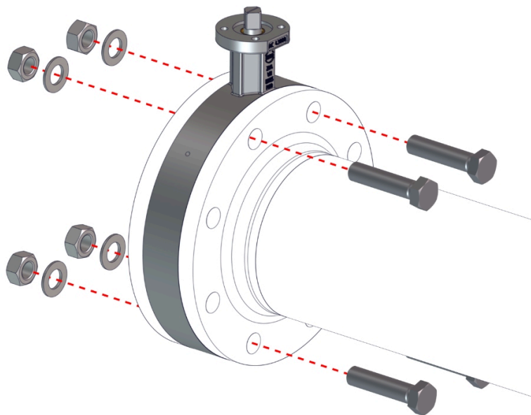
Fig. 8: Posizionamento valvola a farfalla a flangia piena
