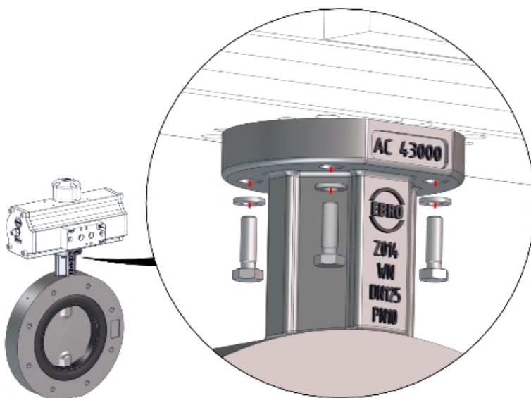
Fig. 7: Principio di montaggio dei componenti
