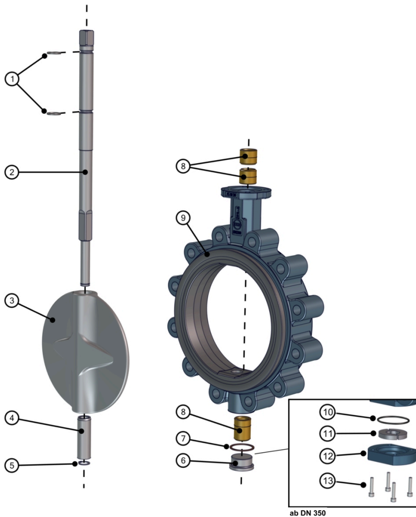
Fig. 16: Distinta base albero TS 2014-B
