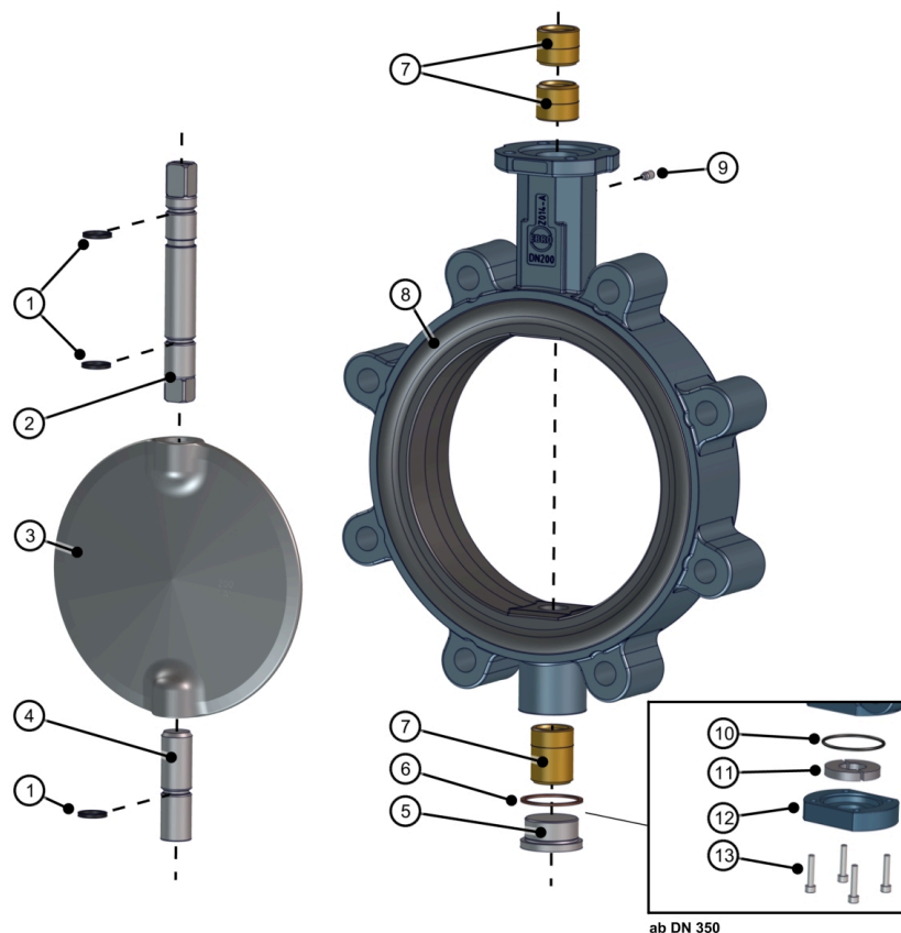
Fig. 15: Distinta base Z014-B
