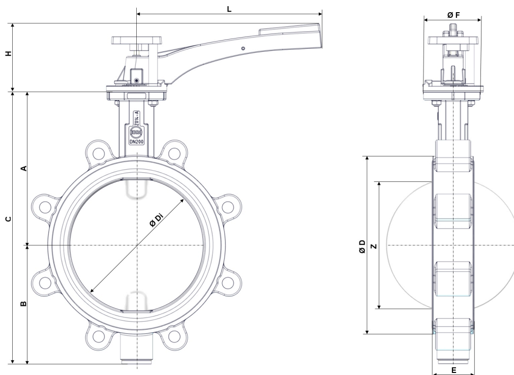
Fig. 3: Dimensioni principali Z104-A THERM
