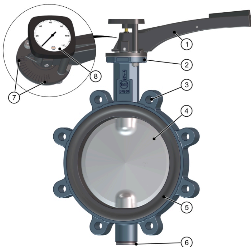
Fig. 2: Componenti
