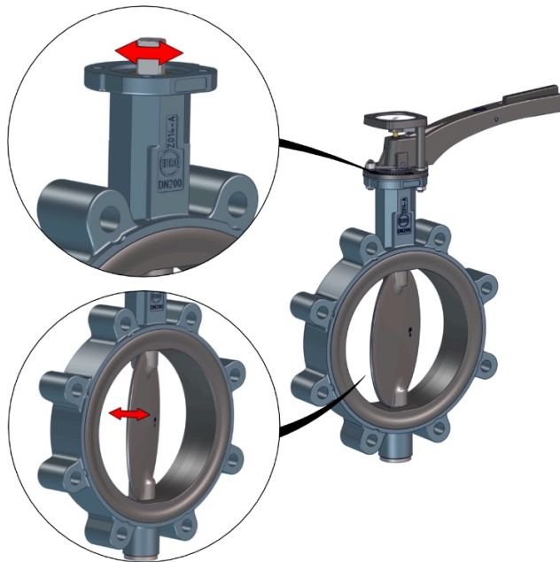
Fig. 4: Parti mobili
