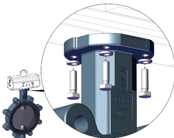
Fig. 7: Principio di montaggio dei componenti
