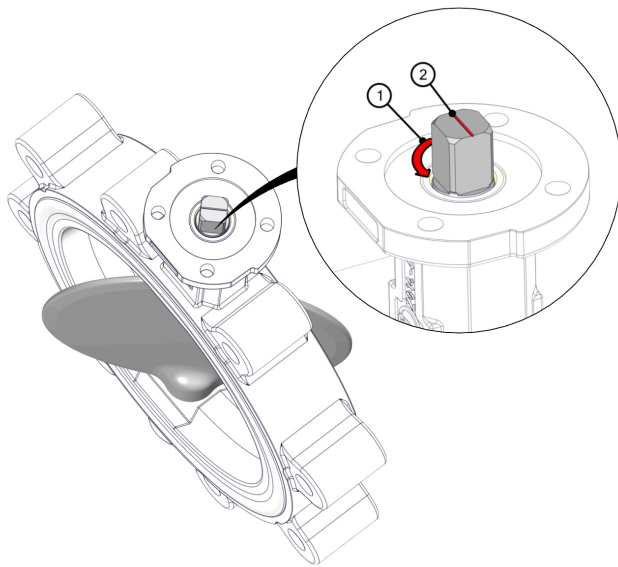
Fig. 14: Direzione di azionamento
