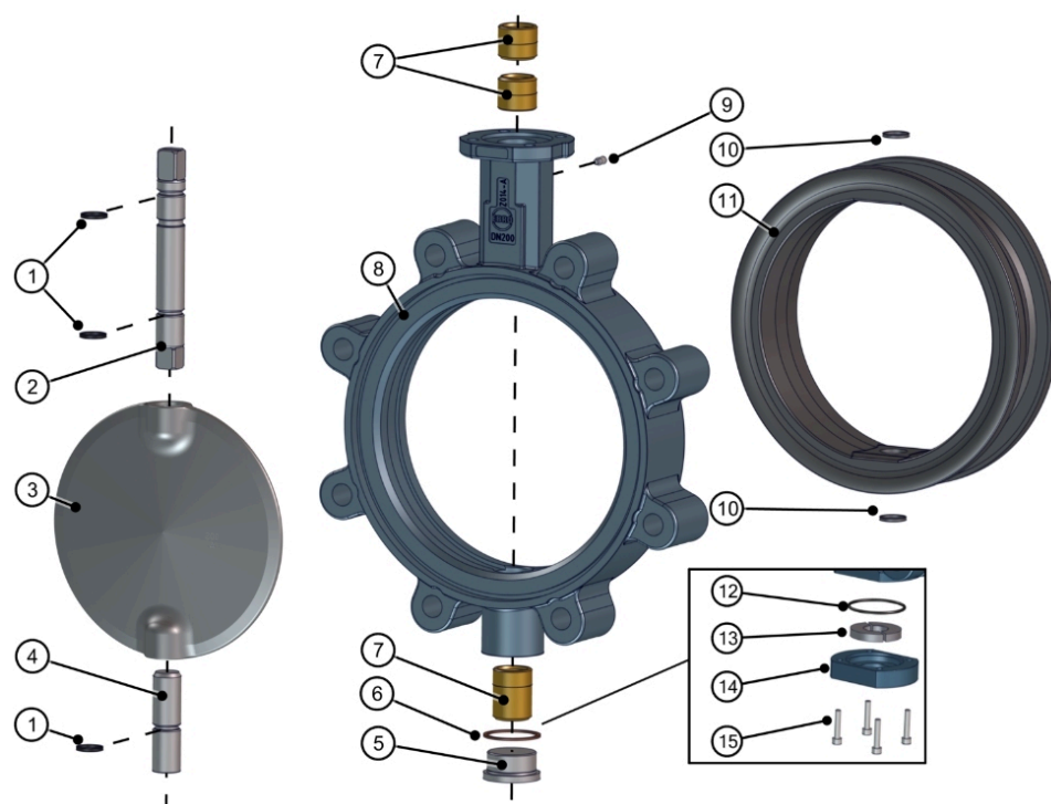
Fig. 15: Distinta base Z14-A
