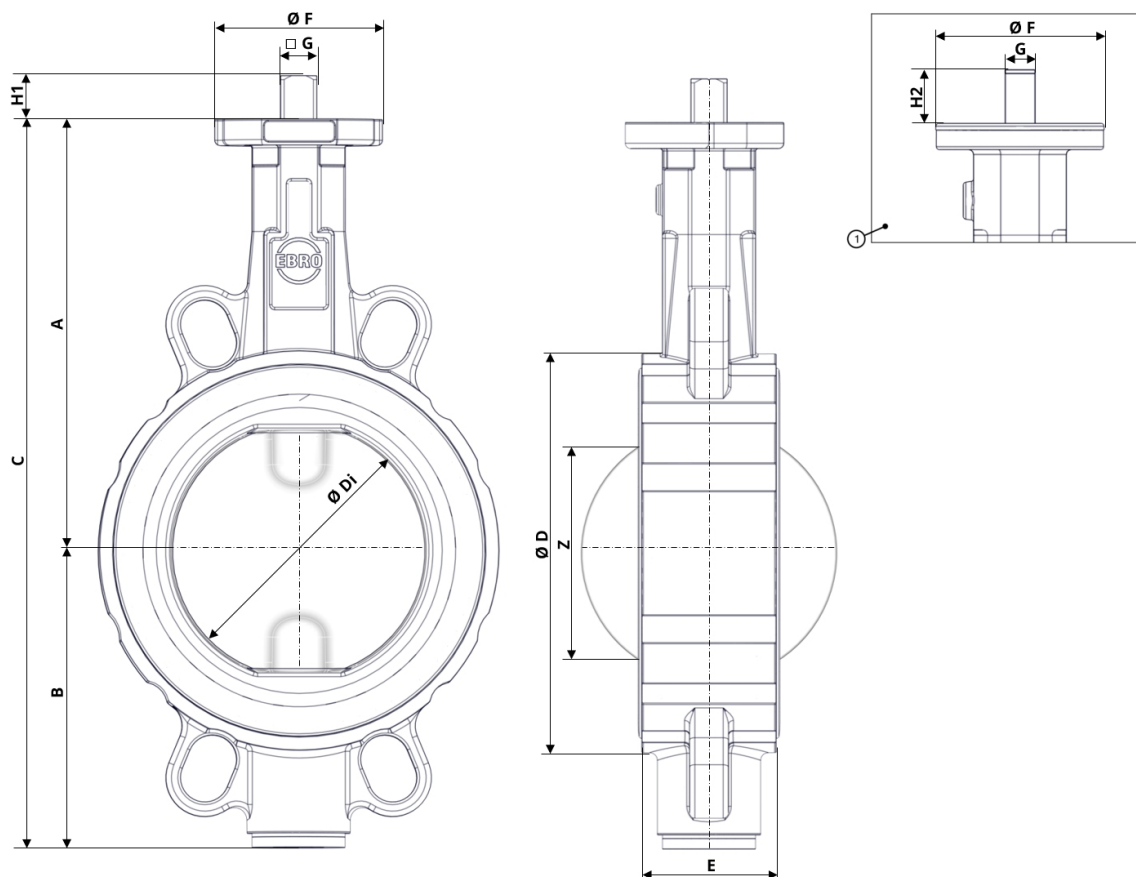
Fig. 3: Dimensioni principali Z011-A
