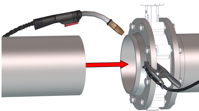
Ábra 10: A cső és a karima összehegesztése
