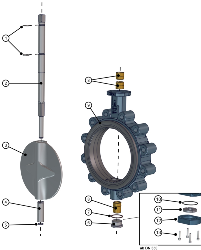
Ábra 16: Darabjegyzék 2014-B, TS-tengely
