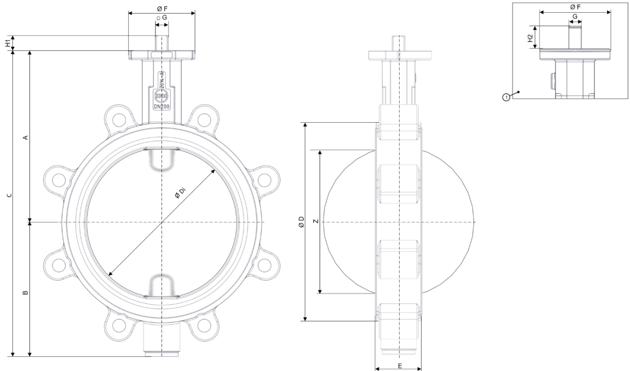
Ábra 3: Fő méretek, Z014-B
