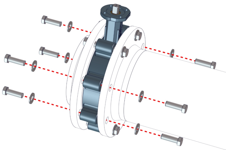
Ábra 9: A karimák közé építhető pillangószelep (LUG) összecsavározása
