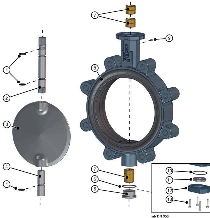
Ábra 15: Darabjegyzék Z014-B
