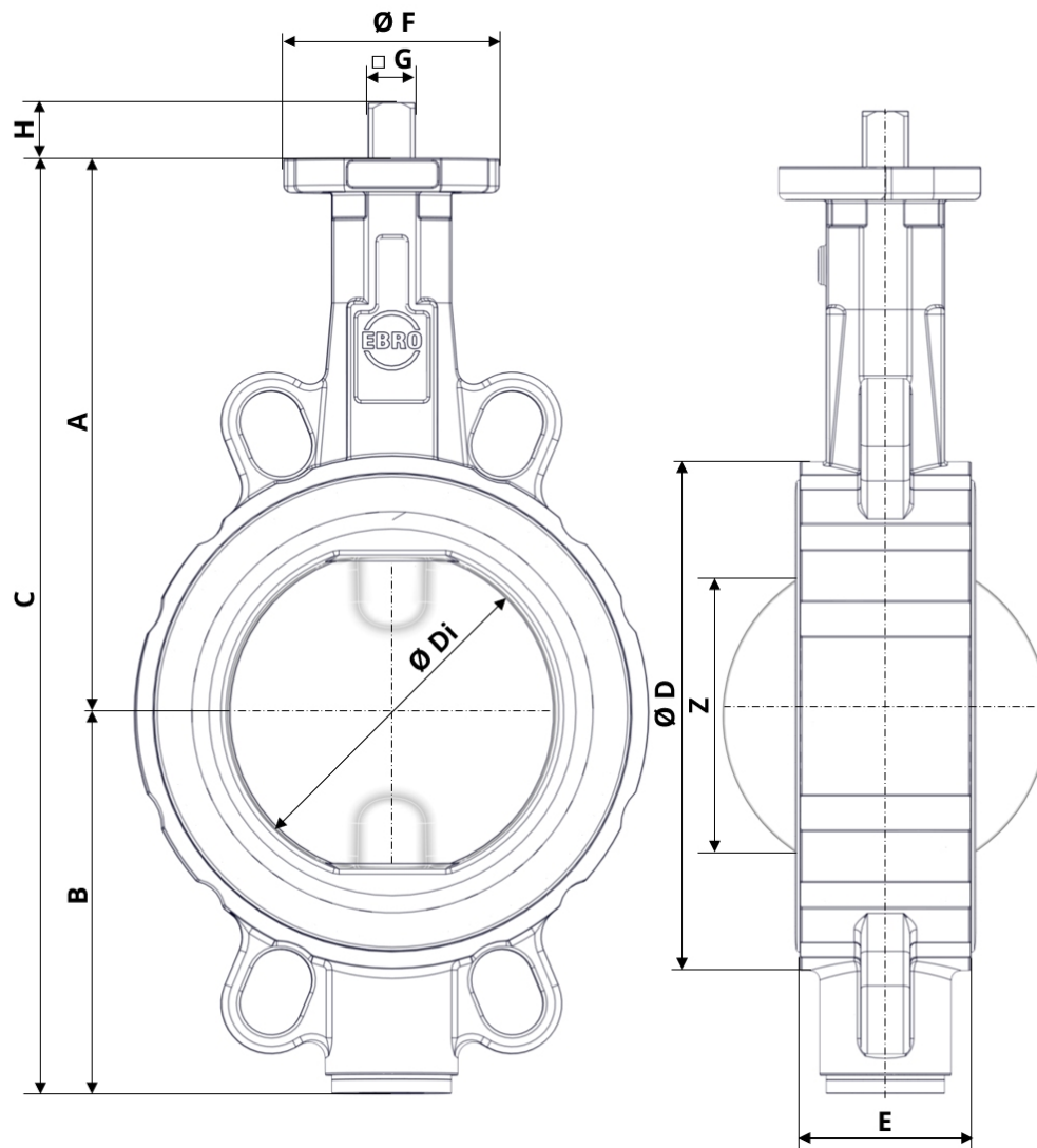
Ábra 3: Fő méretek, Z011-B
