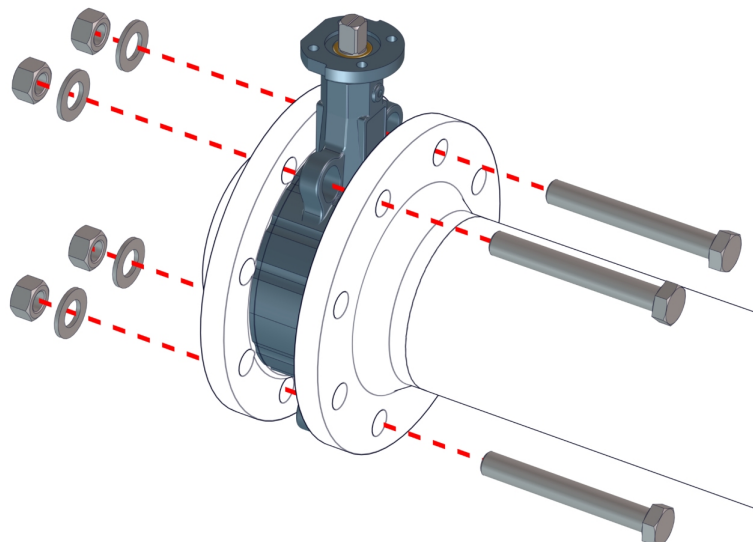
Ábra 8: A karimák közé építhető pillangószelep (WAFER) pozicionálása
