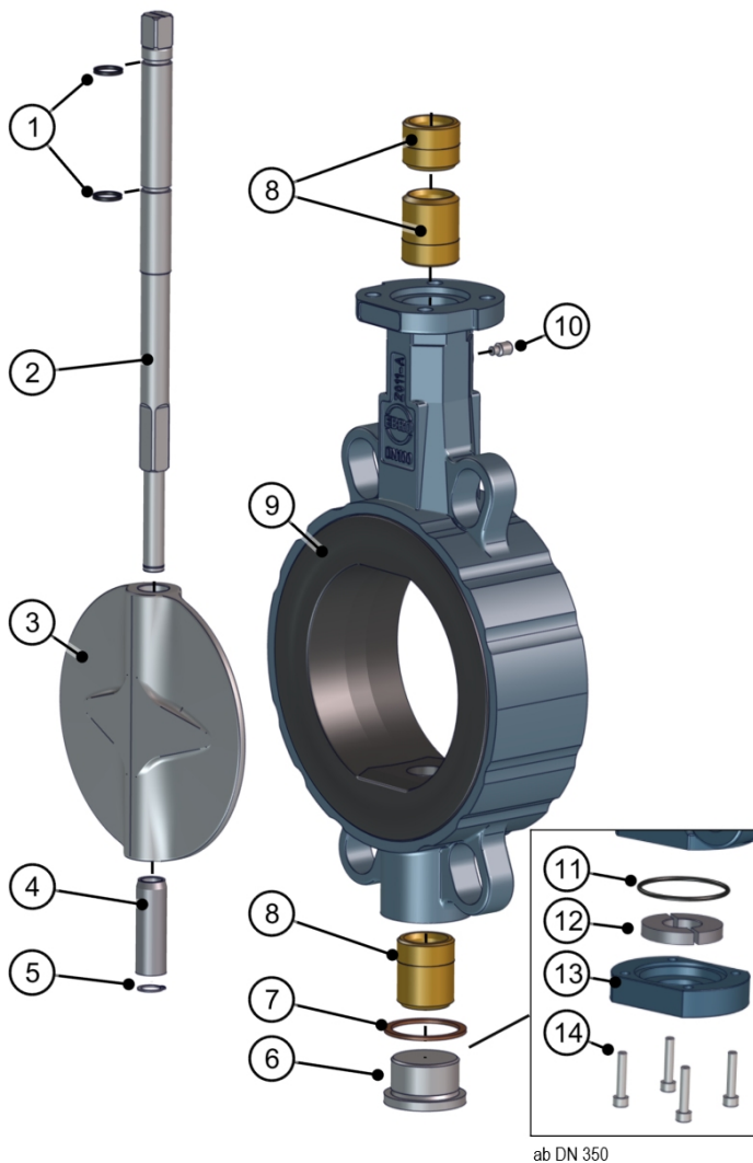
Ábra 16: Darabjegyzék, Z011-B, TS-tengely
