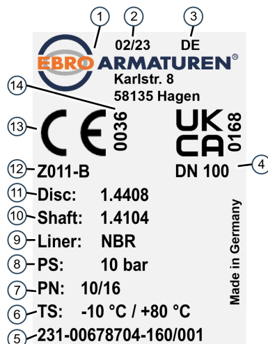
Ábra 1: Példa-típustábla
