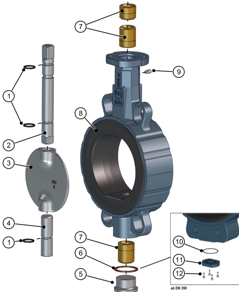
Ábra 15: Darabjegyzék, Z011-B, osztott tengely
