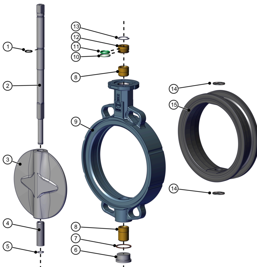
Ábra 18: Darabjegyzék TS pillangószelep-tárcsa 1 tengelyes
