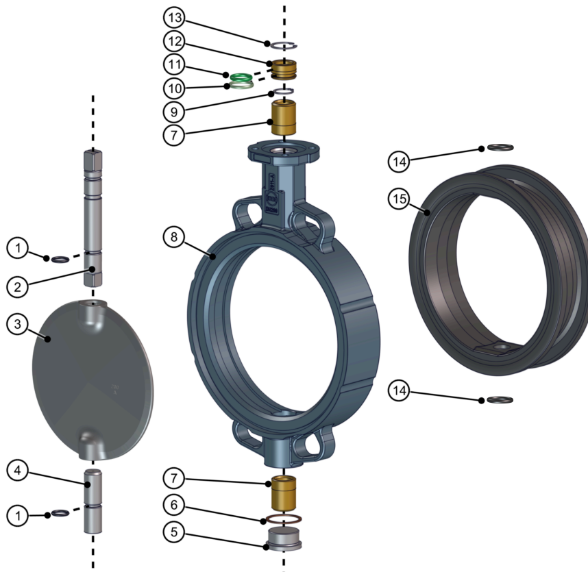
Ábra 17: Darabjegyzék finomöntvény tárcsa 2 tengelyes
