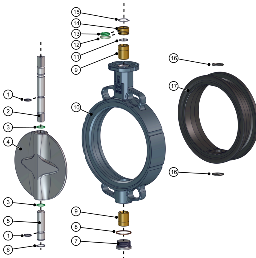
Ábra 19: Darabjegyzék TS pillangószelep-tárcsa 2 tengelyes
