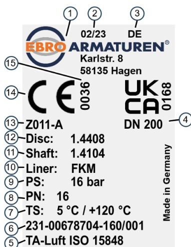
Ábra 1: Példa-típus tábla
