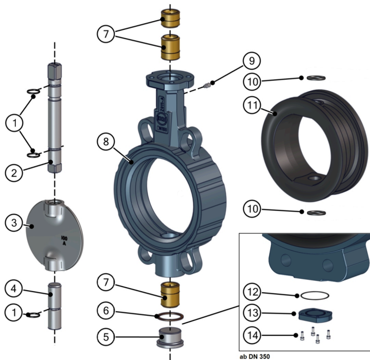
Ábra 15: Darabjegyzék Z011-A osztott tengely
