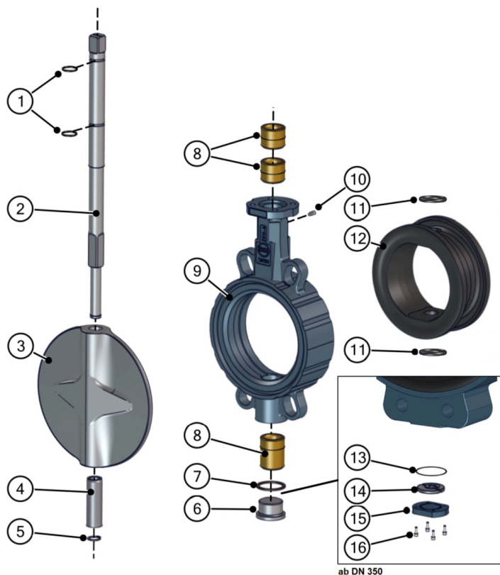
Ábra 16: Darabjegyzék Z011-A TS-tengely
