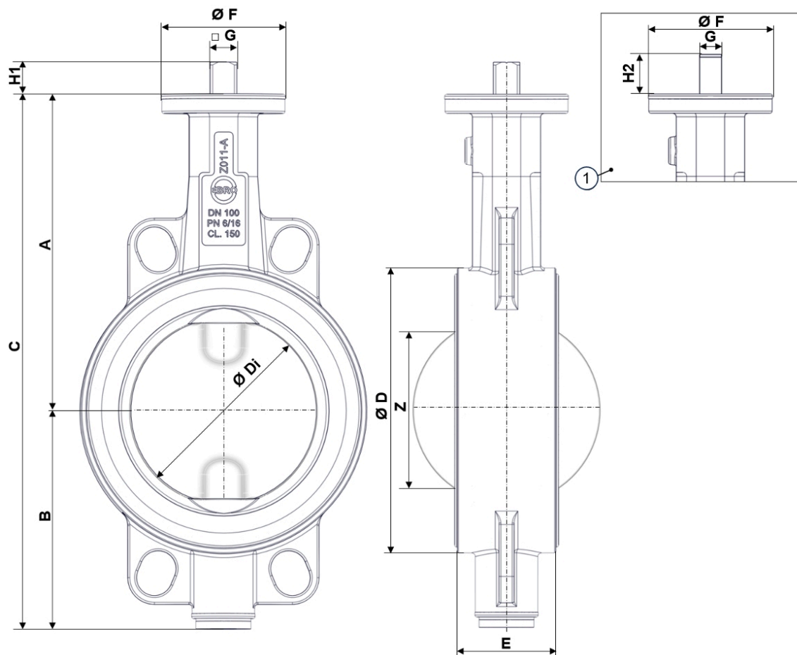
Ábra 3: Fő méretek, Z011-AS
