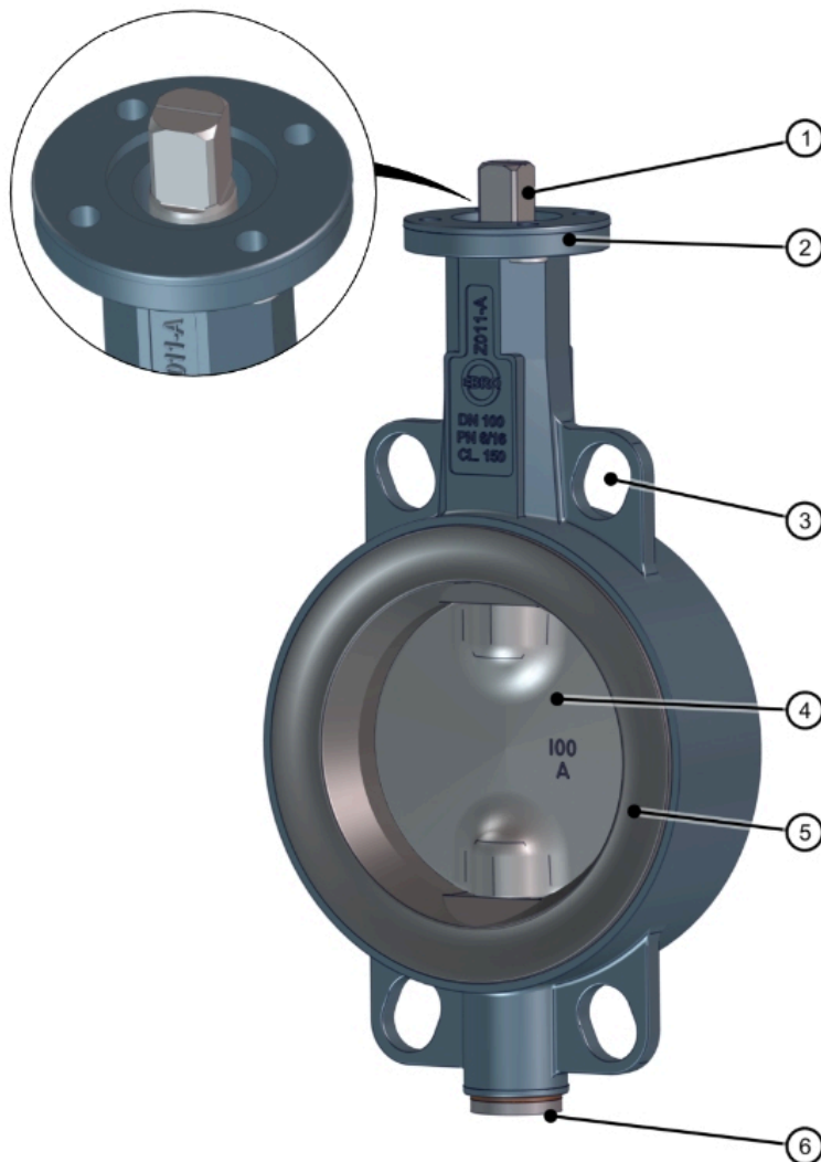
Ábra 2: Komponensek
