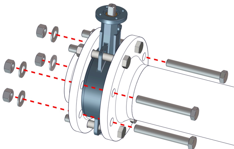
Ábra 9: A karimák közé építhető pillangószelep (WAFER) összecsavarozása
