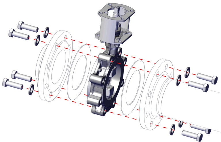
Σχ. 8: Τοποθέτηση βαλβίδας πεταλούδας τύπου lug
