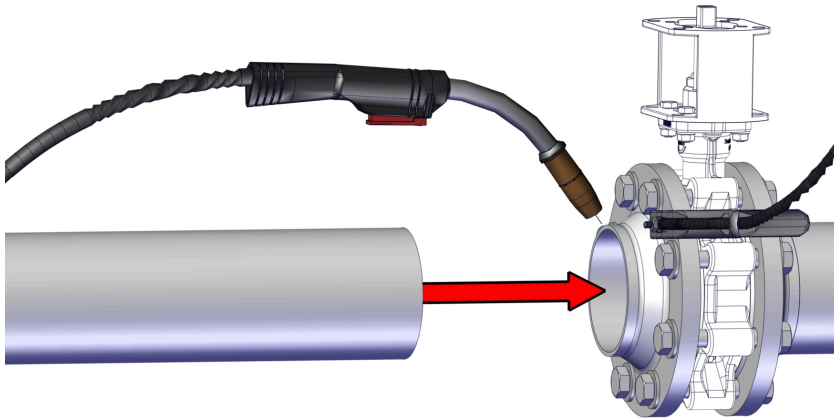
Σχ. 10: Συγκολλήστε τον σωλήνα με τη φλάντζα
