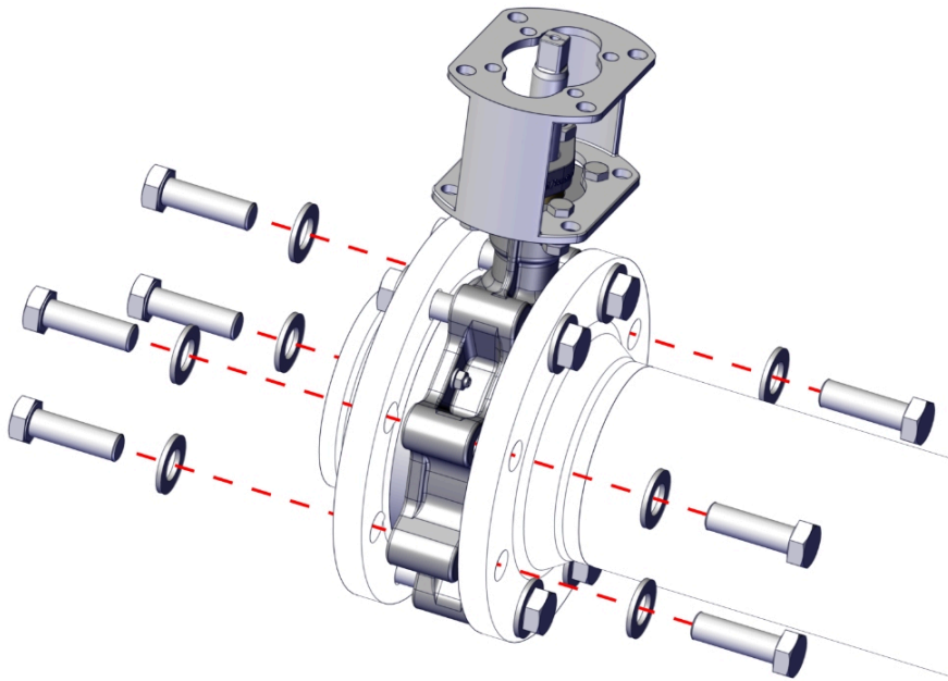
Σχ. 9: Βιδώστε τη βαλβίδα πεταλούδας τύπου lug
