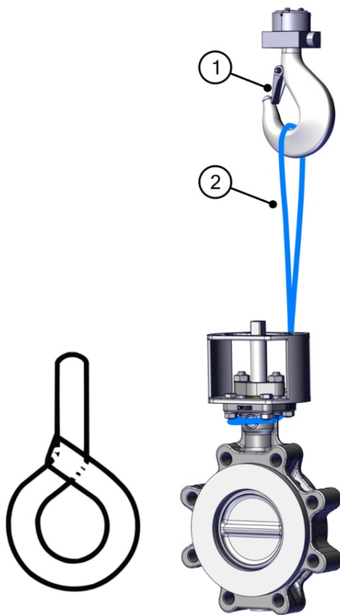
Σχ. 6: Ανύψωση βαλβίδας πεταλούδας τύπου lug
