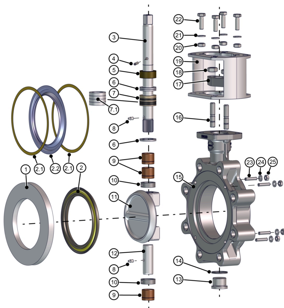
Σχ. 15: Λίστα ανταλλακτικών HP114-HF
