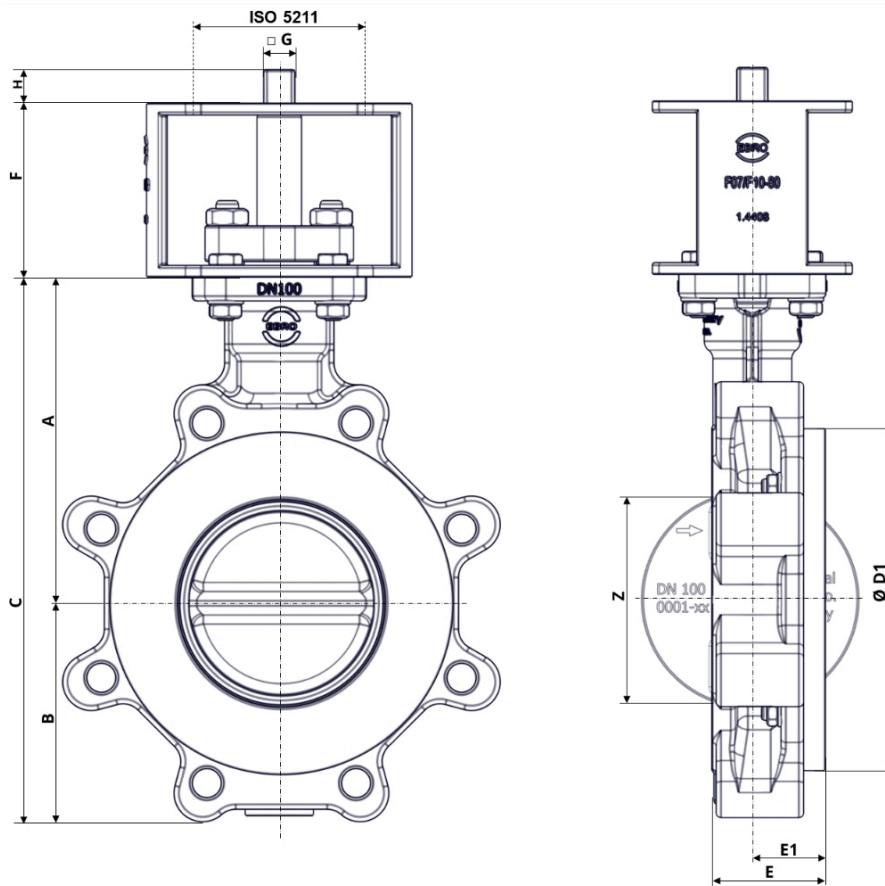
Σχ. 3: Κύριες διαστάσεις HP114-HF
