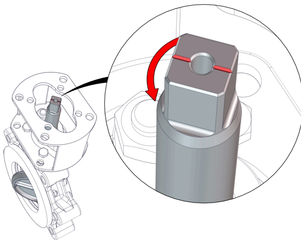
Σχ. 14: Κατεύθυνση ενεργοποίησης
