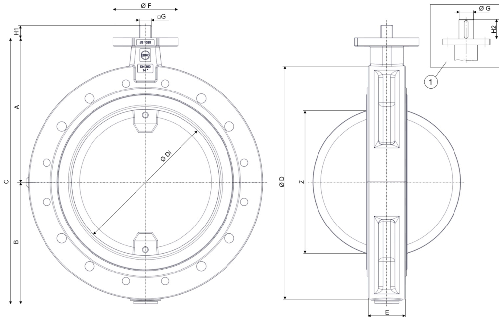
Σχ. 3: Κύριες διαστάσεις T212-A
