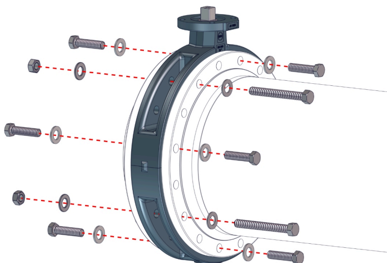
Σχ. 8: Τοποθέτηση βαλβίδα πεταλούδας διπλής φλάντζας
