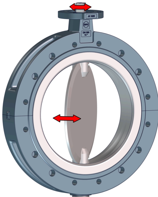
Σχ. 4: Κινούμενα μέρη
