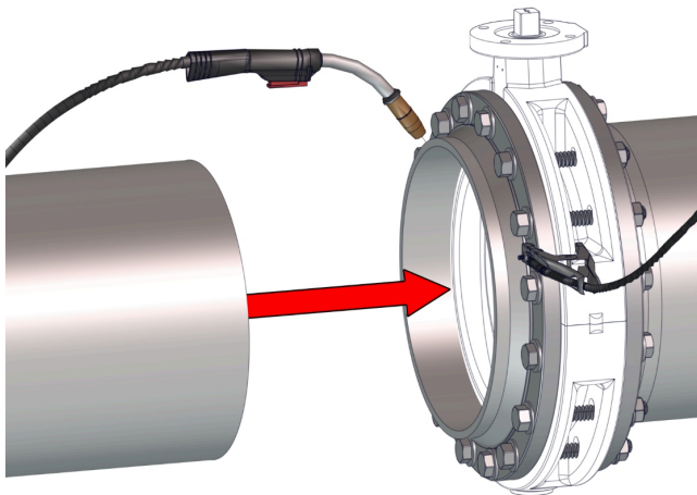
Σχ. 10: Συγκολλήστε τον σωλήνα με τη φλάντζα
