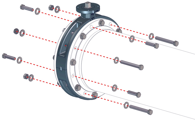
Σχ. 9: Βιδώστε τη βαλβίδα πεταλούδας διπλής φλάντζας
