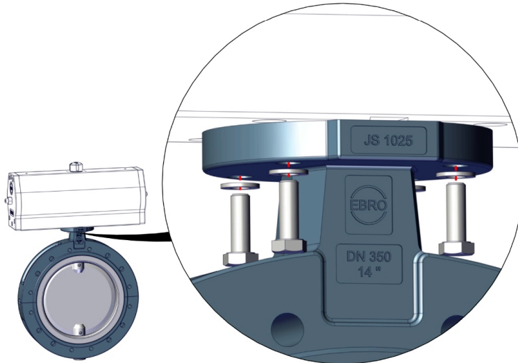
Σχ. 7: Αρχή συναρμολόγησης εξαρτημάτων
