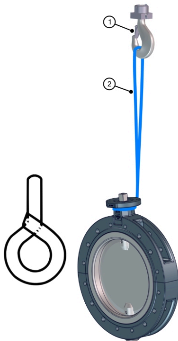
Σχ. 6: Ανύψωση βαλβίδας πεταλούδας διπλής φλάντζας
